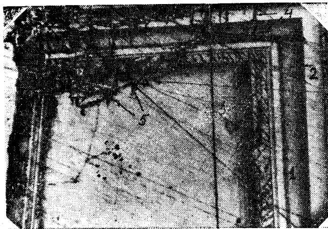
Рис. 1. Зонарный кристалл магнетита в сечении [001] : 1 — плотная часть зоны; 2 — пористая часть зоны; 3 — трещинки в пределах зоны параллельны (111) и (\bar{1}\bar{1}1) ; 4 — трещинки параллельные (101) и (011) ; 5 — игольчатый гематит. Тайгажир (горная Шория) Увел. 60.
