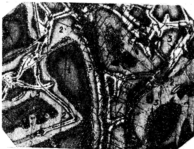
Рис. 7б. Мартитизация магнетита. 1 — реликты первичного магнетита; 2 — плотный магнетит; 3 — гематит; 4 — четко игольчатый гематит. Дашкесан. Увел. 400.
