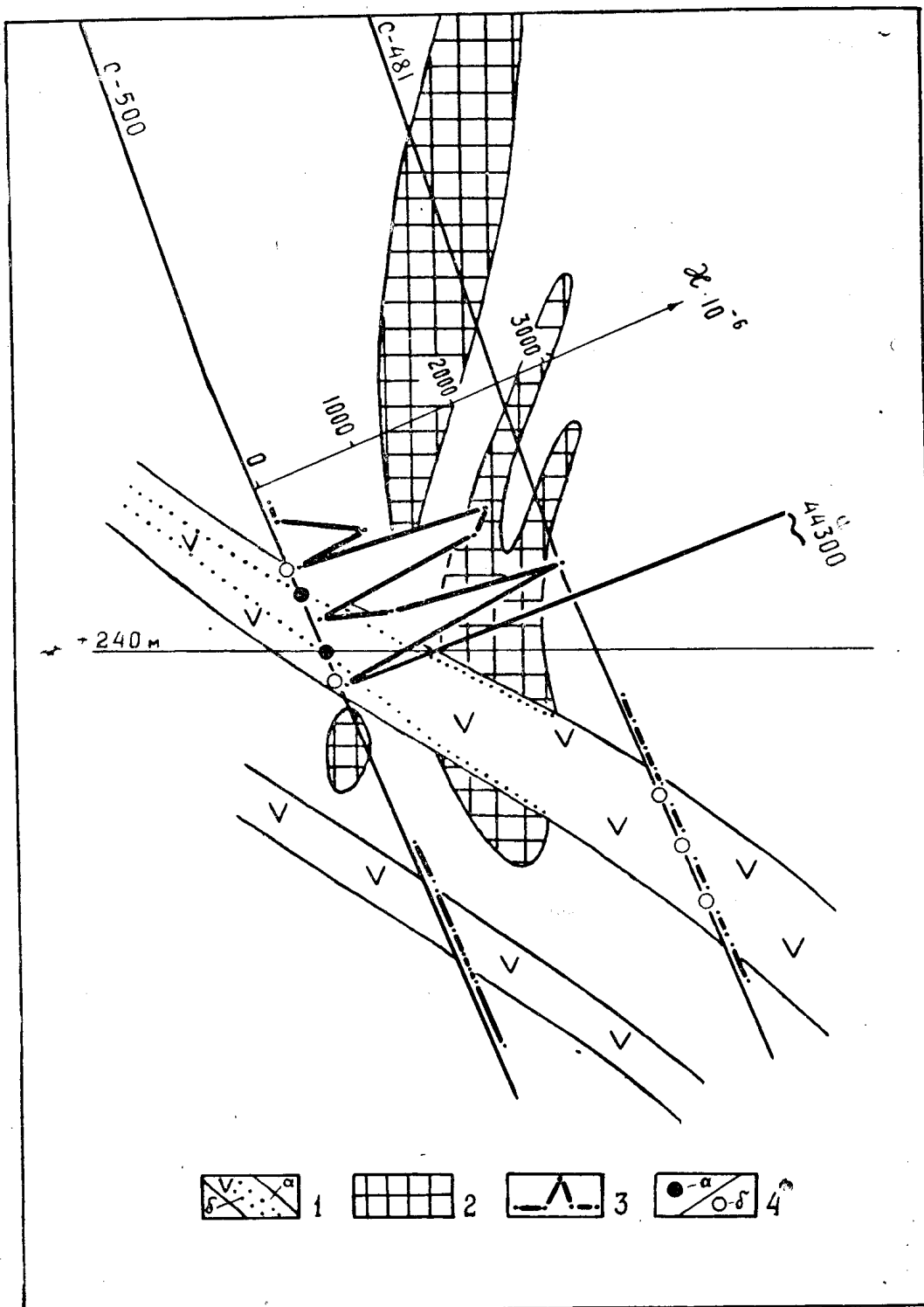
Рис. 1. Ксеногенные струи в дайке диабазового порфирита, секущей магнетитовое рудное тело. Месторождение Северной Аргыштаг. 1—дайки диабазового порфирита (а) и ксеногенные струи (б), 2—магнетитовая руда, 3—графики магнитной восприимчивости, 4—вкрапленность магнетита (а) и лейкоксенизированного ильменита (б).
