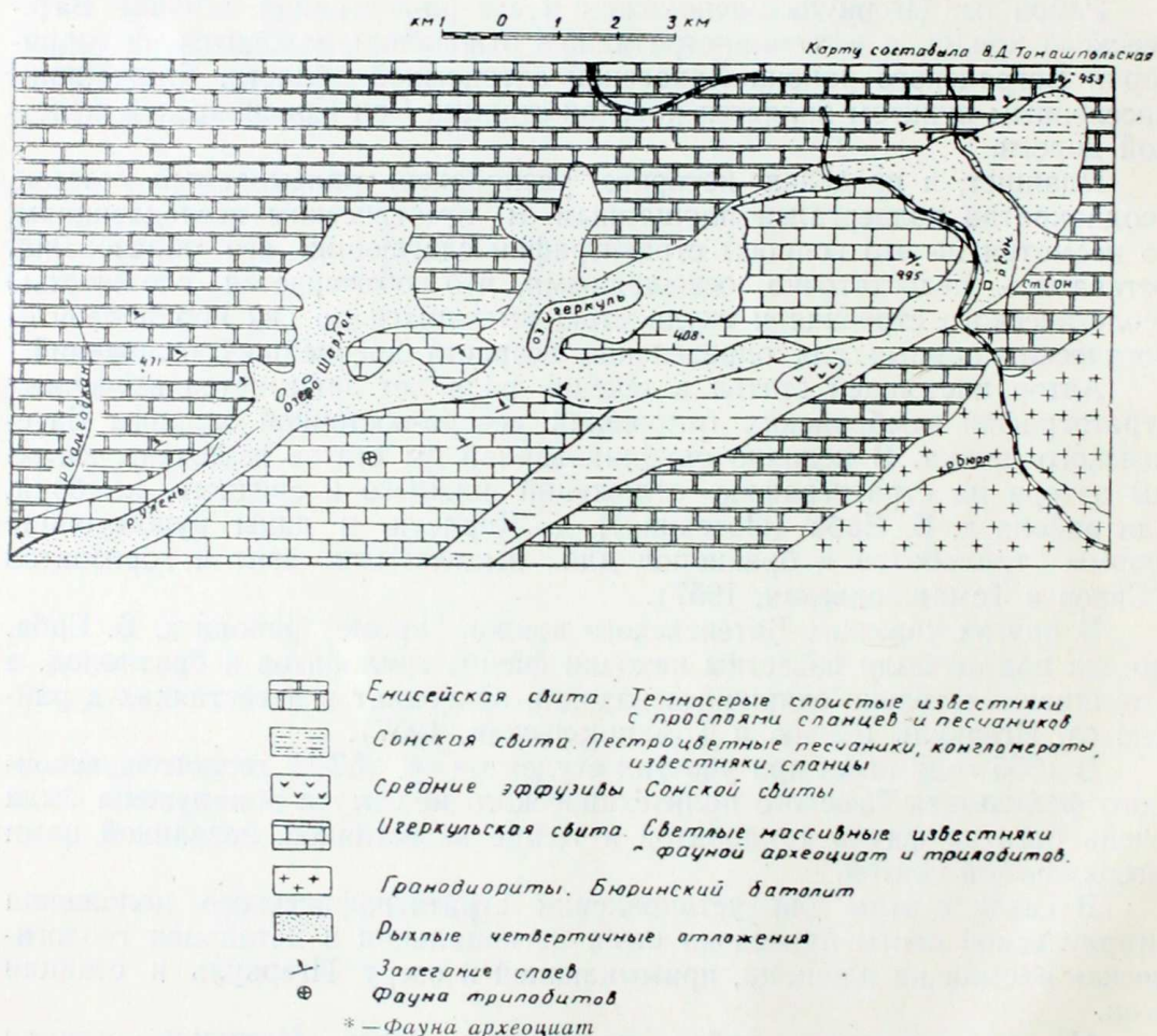
Рис. 1. Схематическая геологическая карта участка оз. Iгеркуль — ст. Сон.
