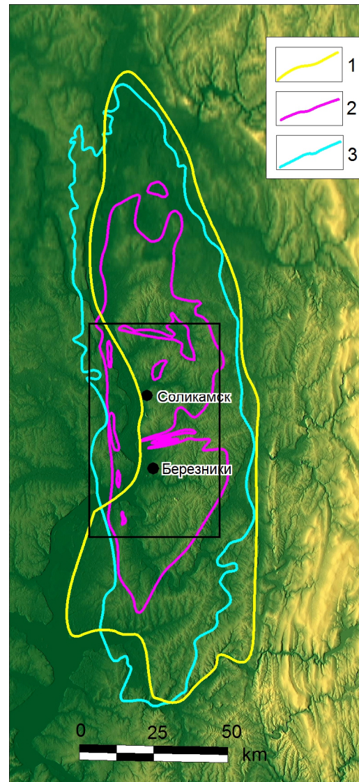
Рис. 1. Соотношение новейшего Соликамского поднятия с соляной линзой и контуром ВКМКС. 1 – контур Соликамского новейшего поднятия, 2 – площадь распространения калийно-магниевых солей (ВКМКС) нижнепермского возраста, 3 – контур соляной нижнепермской линзы, соответствующей Соликамской впадине герцинского возраста. Прямоугольником показана территория исследования
