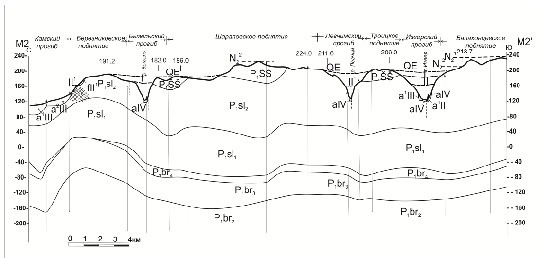
Рис. 5. Геолого-геоморфологический разрез по линии M2-M2'
