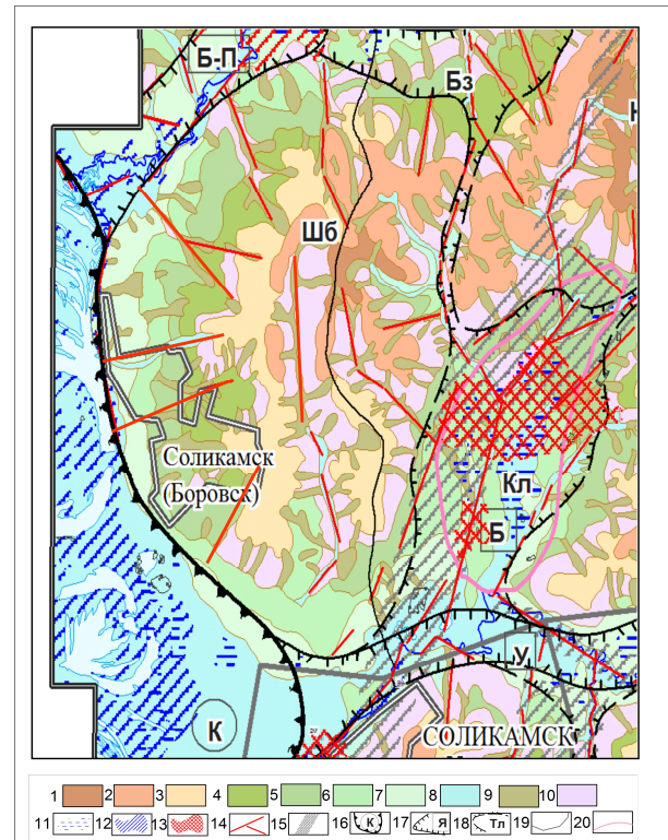
Рис. 3. Фрагмент структурно-геоморфологической карты (Шубинское поднятие). Формы рельефа (денудационный 1 – плиоценовая, 2 – эоплейстоценовая, 3 – раннеоплейстоценовая ступени); флювиогляциальный (4 – 4-я терраса (долинный зандр)); аллювиальный (5 – 3-я терраса, 6 – 2-я терраса, 7 – 1-я терраса, 8 – пойма; 9 – днища оврагов, балок, ложбин; 10 – склоны водоразделов, речных долин и оврагов, не расчлененных по возрасту). Экзогенные процессы: 11 – заболачивание, 12 – участки периодического затопления паводками, 13 – участки возможной инфильтрации поверхностных вод в сильвинит-карналлитовую зону из-за отсутствия на ней ПКС.
