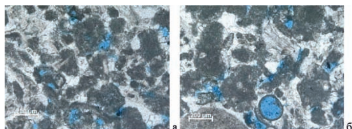
Рис. 11. Известняк сферо-узорчатый, водорослевый спаритовый. Николи: параллельные (а, б)
