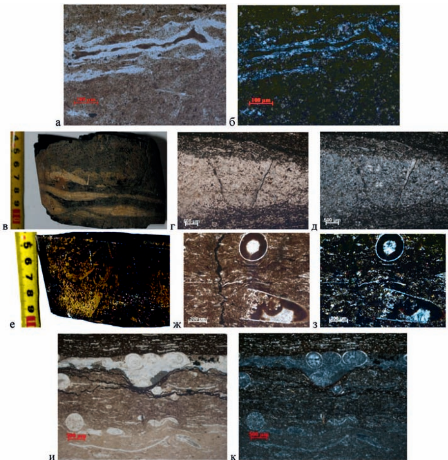
Рис. 2. Пористость, не связанная со структурой и выполненная битумоидами в высокоуглеродистых породах: а-б) микро «каверны» в кремневых высокоуглеродистых ритмитах; в) линзы шламового известняка, трещиноватого (фото образца); г-з) трещины, заполненные битумоидами (е-фото образца кремневого ритмита трещиноватого); и-к) микростилолитовые швы. Николи: параллельные – а, г, ж, и); скрещенные – б, д, з, к)
