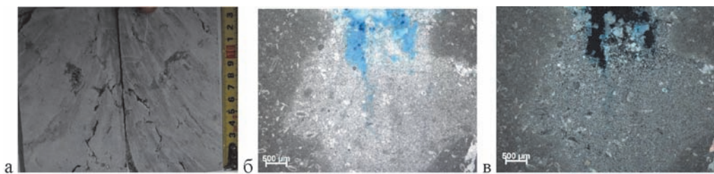
Рис. 9. Известняк криптозернистый с примесью ракушнякового шлама, биокластов нефтенасыщенный, с мелкими кавернами, ориентированными, преимущественно, параллельно слоистости (а-в). Николи: б) параллельные; в) скрещенные
