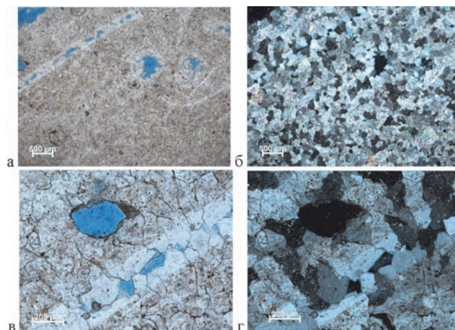
Рис. 7. Доломит средне-мелкозернистый. а-г) Реликтовые биокласты; а-г) пустоты приуроченные к биокластам и основной массе. Никели: параллельные (а, в); скрещенные (б, г).
