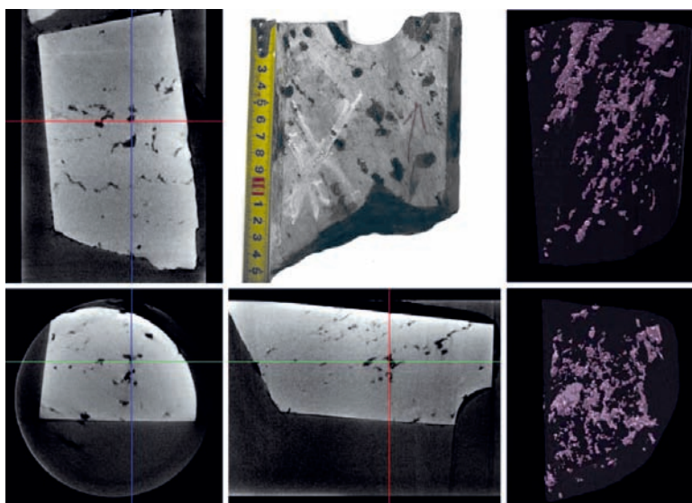
Рис. 8. Ортогональные рентгеновские сечения образца известняка и стереологические модели (справа) пустотного пространства. Съёмка полно-размерных образцов ядра проводилась на томографе РКТ-180-1
