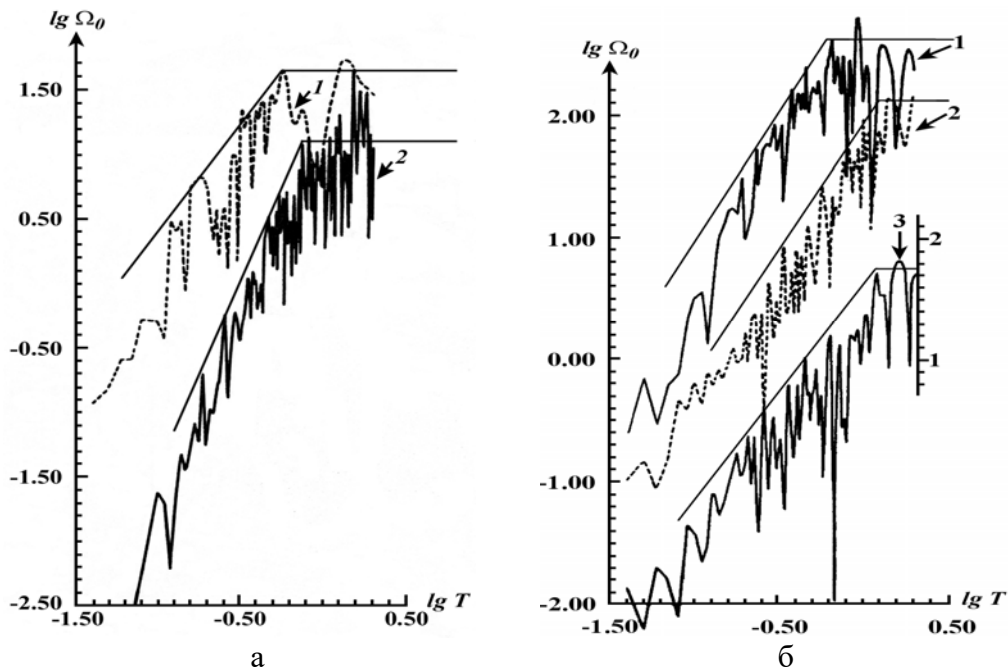
Рис. 2. Амплитудные спектры поперечных волн ощутимых землетрясений 1990 г. по [3]: а – 2 июля в 0^{\text{h}}35^{\text{m}}50.9^{\text{s}} по записям сейсмических станций: 1– ALU, 2– KZN; б – 16 августа в 04^{\text{h}}32^{\text{m}}18.3^{\text{s}} по записям: 1– ALU, 2– SIM, 3 – YAL. Прямыми линиями показана авторская аппроксимация спектров в рамках модели Брюна.
