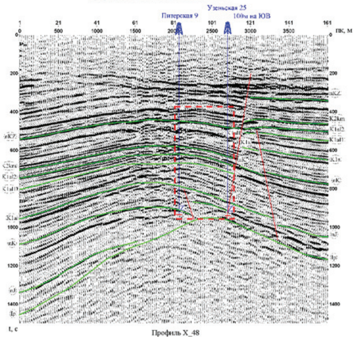
Рис.3. Комплексирование электроразведки и сейсморазведки на Узеньском месторождении
