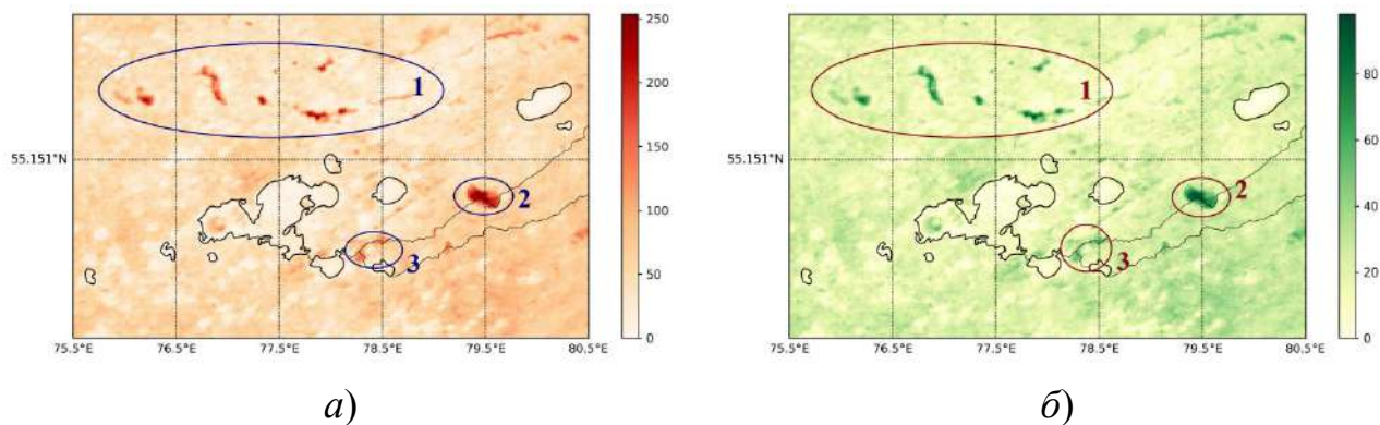
Рис. 2. а) накопительная сумма аномальных значений индекса за 2001–2015 гг.; б) количество пикселей, в которых значение индекса превышает пороговое значение за 2001–2015 гг.
