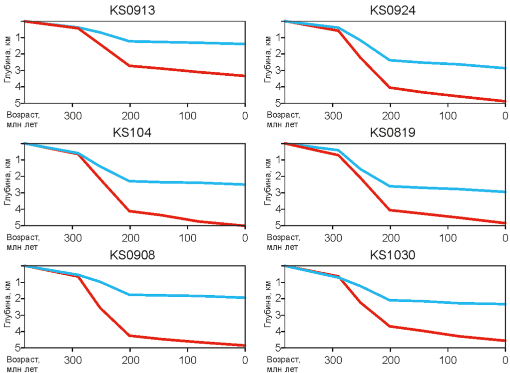
Рис. 5. Кривые тектонического прогибания, рассчитанные в программе TecMod для шести изучаемых профилей. Для каждого профиля показано тектоническое прогибание, рассчитанное для псевдоскважин (их расположение см. на рис. 4) в наиболее глубокой части бассейна (красная линия) и на его периферии (синяя линия)
