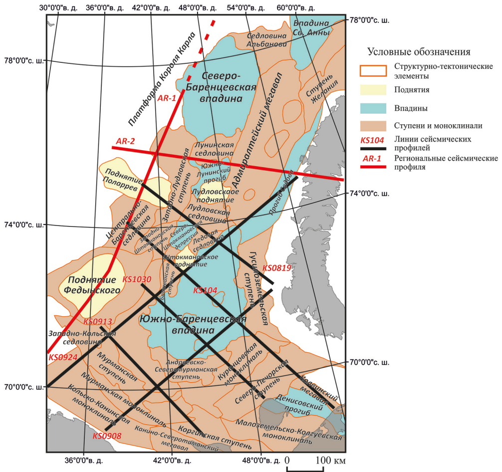
Рис. 1. Тектоническая схема Восточно-Баренцевского осадочного бассейна по (Соболев и др., 2008)
