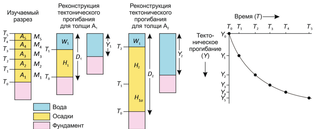
Рис. 2. Последовательность процедур при расчете тектонического погружения по (Bond and Komiz, 1984)
