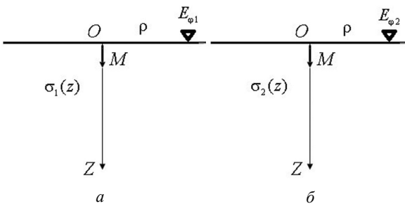
Рис. 1. Геоэлектрические разрезы «1» и «2»
