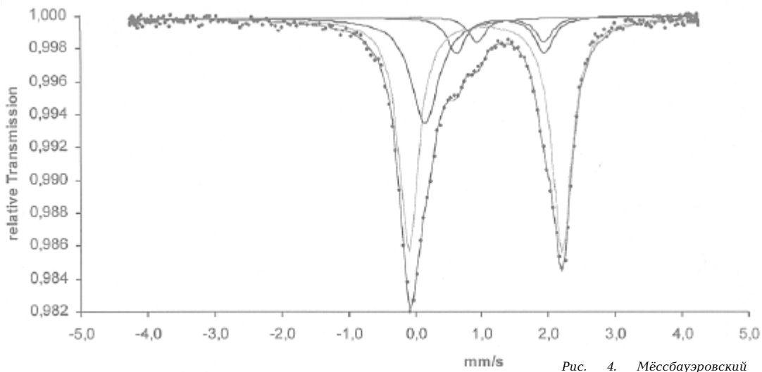
Рис. 4. Мёссбауэровский спектр атенсионта
