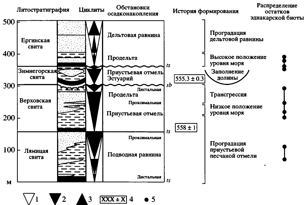
Рис. 4. Строение, обстановки осадконакопления и история формирования отложений вендского комплекса Юго-Восточного Беломорья. Стратиграфические границы: sb – секвентная; ts – трансгрессивная.
