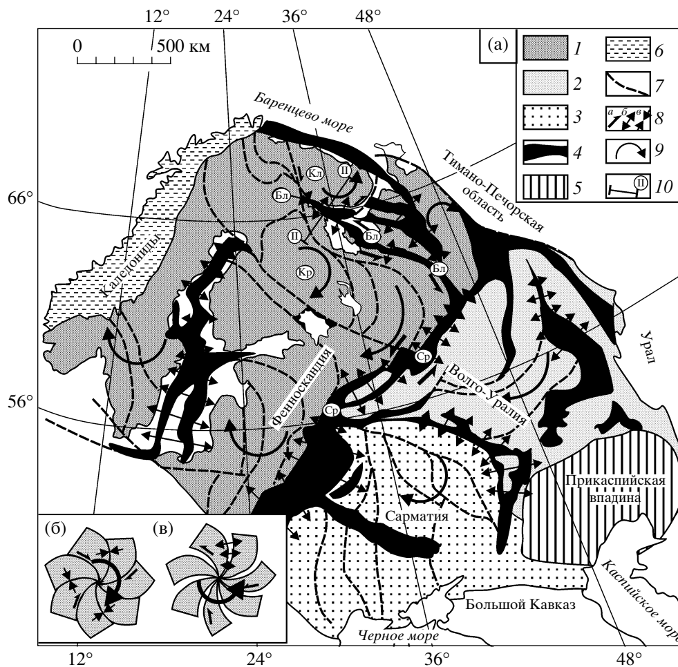
Рис. 1. а – схема тектонической делимости и размещения рифтогенных структур ВЕП (составлена по [1, 6, 7]). б, в – упрощенные модели процессов структурообразования в условиях вращения. 1–3 – главные тектонические единицы фундамента ВЕП: 1 – Фенноскандия, 2 – Волго-Уралья, 3 – Сарматия; 4 – рифтовые системы; 5 – Прикаспийская впадина; 6 – каледониды; 7 – разрывные нарушения; 8 – направления сдвиговых перемещений (а), растяжения (б) и сжатия (в); 9 – направления вращения блоков; 10 – линия геолого-геофизического разреза на рис. 2г. Рифтовые системы: Ср – Среднерусская, Бл – Беломорская. Архейские массивы: Кр – Карельский, Кл – Кольский.
