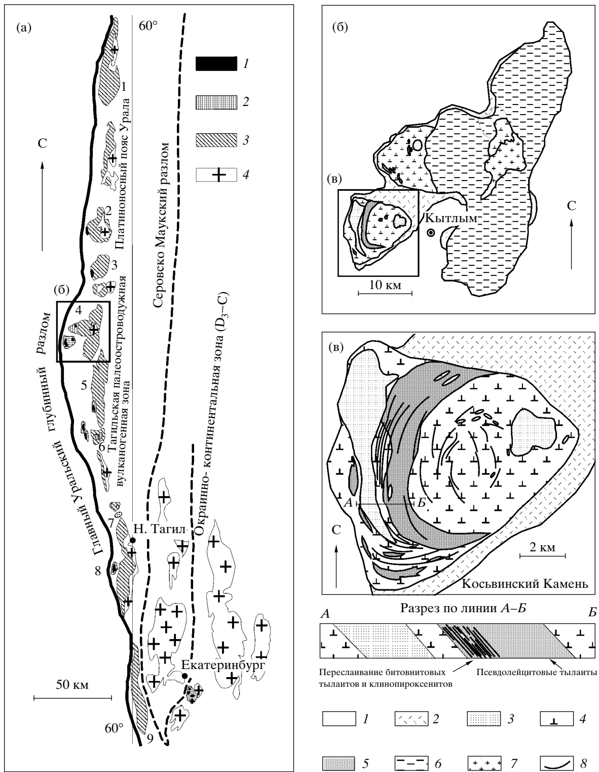
Рис. 1. а – Платиноносный пояс Урала: 1 – дуниты; 2 – верлиты и клинопироксениты; 3 – габброиды; 4 – гранитоиды; цифрами на схеме обозначены наиболее крупные массивы: 1 – Чистопский, 2 – Денежкин Камень, 3 – Кумбинский, 4 – Кытлымский, 5 – Павдинский, 6 – Качканарский, 7 – Тагило-Бараңчинский, 8 – Нижнетагильский, 9 – Ревдинский. Схемы геологического строения Кытлымского массива (б) и горы Косьвинский Камень (в) [2], упрощенные нами: 1 – вмещающие аповулканогенные породы, 2 – кытлымиты, экзоконтактные пироксеновые роговики, 3 – дуниты, 4 – клинопироксениты, 5 – тылаиты нерасчлененные, битовнитовые и псевдолейцитовые, 6 – габбро-нориты и оливиновые габбро, 7 – гранитоиды, 8 – ориентировка полосчатости и гнейсовидности в породах.
