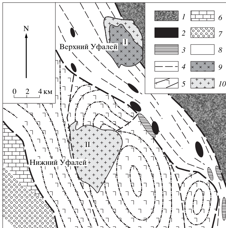
Рис. 1. Схематическая геологическая карта Уфалейской зоны (по К.С. Иванову, 1999): 1 – породы зоны ГУГР: углито-кварцевые сланцы, филлиты, базальтовые порфириды ( O_{2-3} ); Восточно-Уфалейская зона (высокобарическая): 2 – амфиболиты ( S-D_1 ), 3 – метасульфиды ( S-D_1 ), 4 – милониты; Западно-Уфалейская зона: 5 – гнейсы и амфиболиты ( Pt_2 ); 6 – известняки ( D_2 ); 7 – толщи чехла Русской платформы ( Pz ); 8 – Тараташский комплекс; 9 – диориты; 10 – гранодиориты и граниты. Массивы: I – Суховязовский, II – Нижнеуфалейский.
