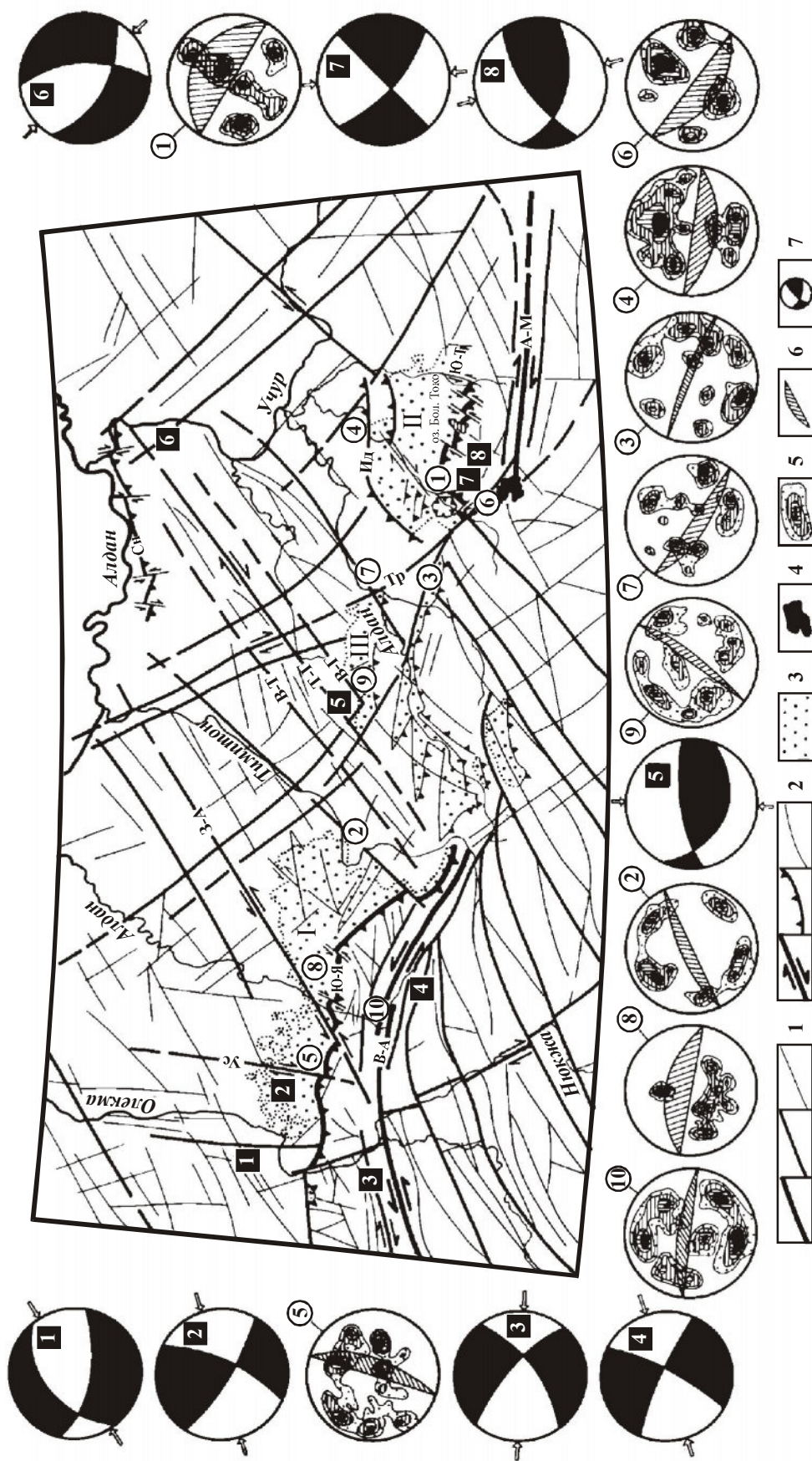
Рис. 7. Схема активных разломов Южной Якутии.
