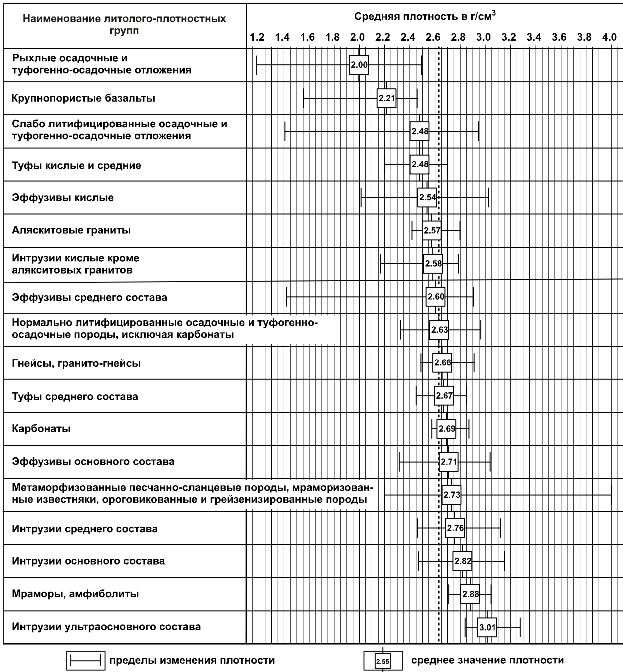
Рис. 4. Сводный литолого-плотностной ряд горных пород и осадочных отложений южной части Приморья
