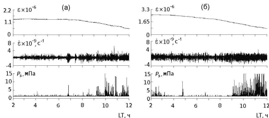
Рис. 5. Примеры аномалий геоакустической эмиссии при сжатии приповерхностных пород 15 (а) и 18 (б) октября 2009 г.; \varepsilon – относительная деформация пород, \dot{\varepsilon} – скорость деформирования, P_s – суммарное за 4 секунды акустическое давление в диапазоне частот 0.6–2.0 кГц.
