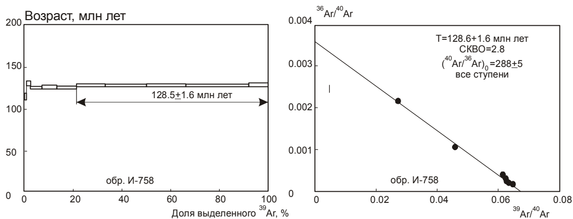
Рис. 2. Графики ступенчатого отжига и корреляционные диаграммы изотопов аргона для серицита из гидротермально-метасоматических образований рудопроявления Десс.
