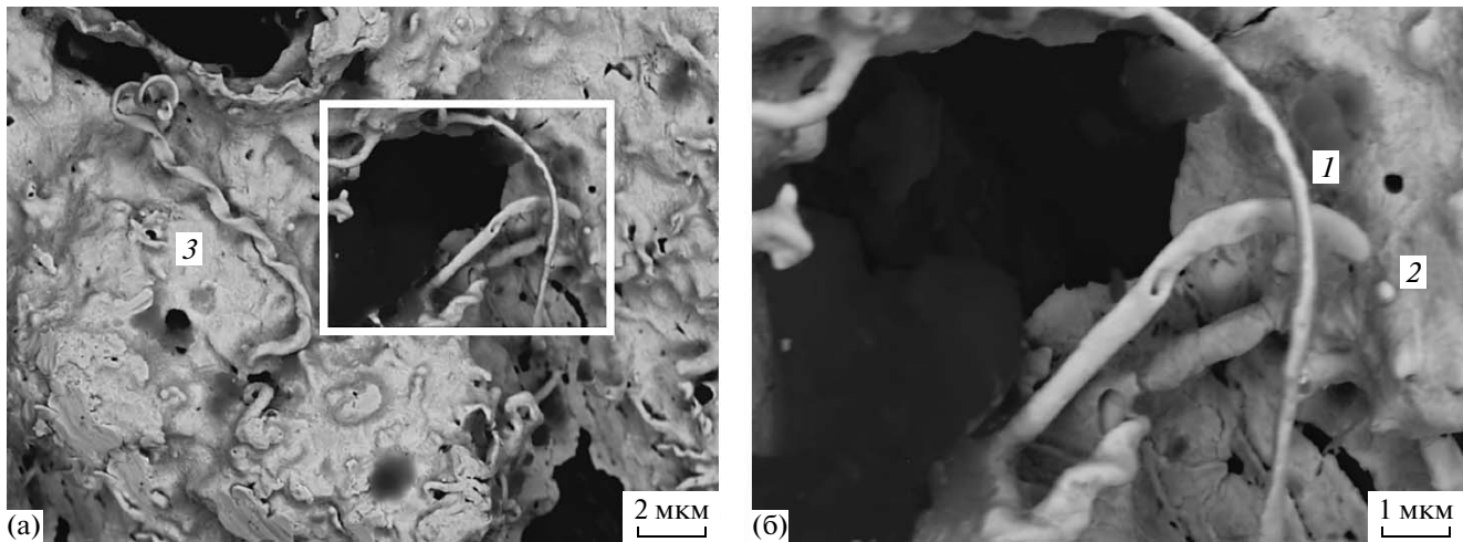
Рис. 3. Нанотрубки (1), наносфероиды (2) и наноспираль (3) золота. Рамкой (а) выделен увеличенный фрагмент наноструктуры (б). Изображение в обратно отраженных электронах.
