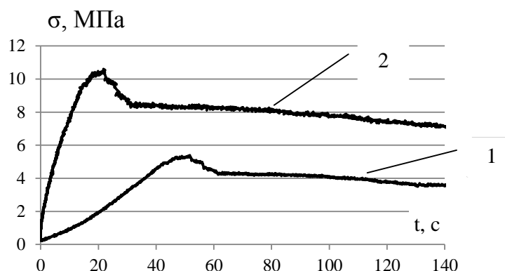
Рис. 2 – Диаграммы напряжение – деформация при одноосном (1) и двухосном сжатии (2); время возникновения трещины t = 130 с при одноосном нагружении, t = 140 с при двухосном нагружении
