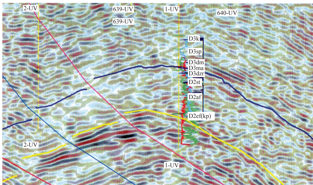
Рис. 4. Фрагмент временного разреза по профилю 796-06
