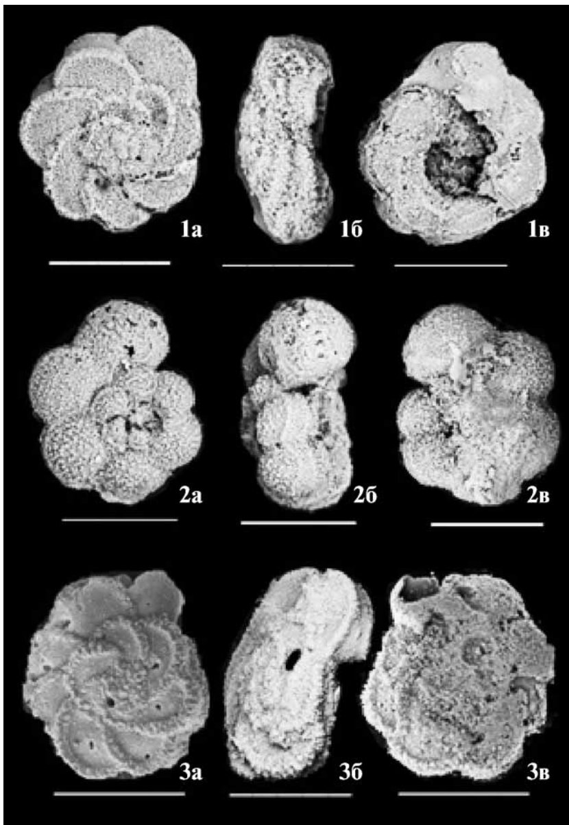
Рис. 8. Планктонные фораминиферы из разреза Алан-Кыр (а — дорзальная сторона, б — периферический край, в — вентральная сторона): 1а–в — Marginotruncana pseudolinneiana Pessagno, образец 13-2-6, верхний сантон; 2а–в — Archaeoglobigerina cretacea (d'Orbigny), образец 13-1-1, верхний коньяк; 3а–в — Marginotruncana coronata (Bolli), образец 13-2-6, верхний сантон. Линейка 250 \mu\text{m}
