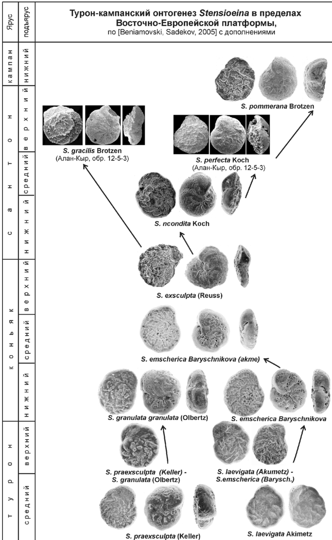
Рис. 6. Stensioeina perfecta Koch и типичные S. gracilis Brotz. — недостающие звенья в развитии стенсиоин в Восточной Европе
