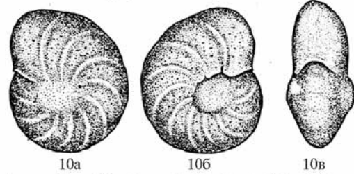
Anomalina (Brotzenella) insignis (Lipnik) [Акимец, 1961; с. 161, т. XV, фиг. 10 а-в], Белоруссия, кампан
