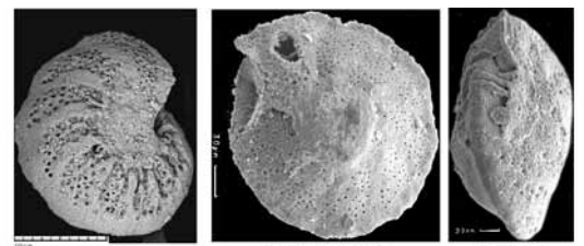
дорзальная (обр. 13-2-6) вентральная (обр. 12-5-3) профиль (обр. 12-5-3)
