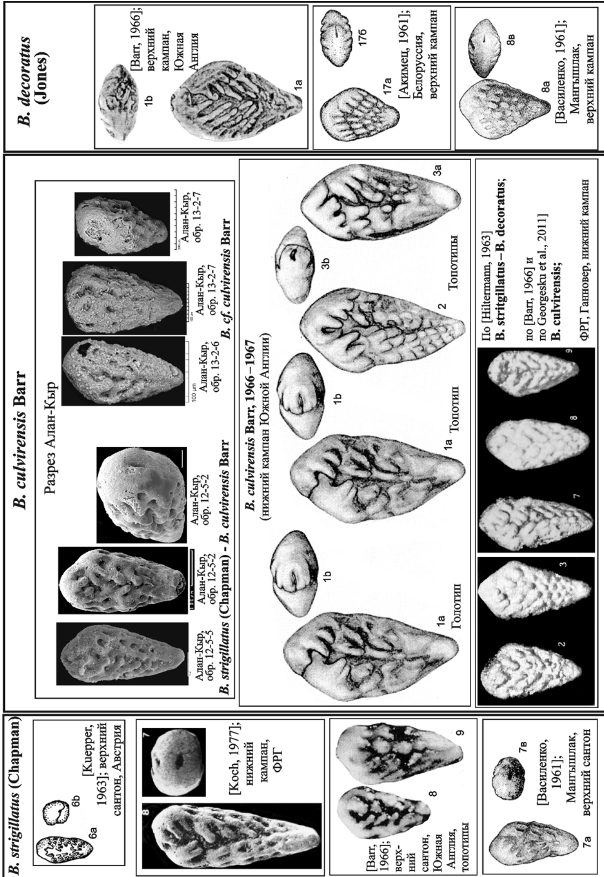
Рис. 3. Три важнейших в стратиграфическом отношении видов рода Bolivinoidea : B. strigillatus (Charman), B. culvirensis Barr и B. decoratus (Jones), играющих большую роль в филологии и зональной стратиграфии верхнего сантона – верхнего кампана различных регионов, а также место изученных представителей Bolivinoidea из разреза Алан-Кыр в таксономии этих трех биливинидесов
