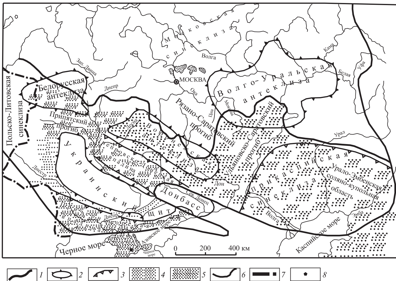
Рис. 10. Биохоремы (биоохории) Anomalinoidea insignis и Cibicides temirensis в восточной части ЕПО и ее крымском обрамлении, границы тектонических структур Восточно-Европейской платформы, по [Найдин и др., 1986]: 1 — ВЕП, 2 — щиты и антеклизы, 3 — синеклизы и впадины; ареалы (биоохоремы); 4 — Anomalinoidea insignis ; 5 — Cibicides temirensis ; 6 — граница современного распространения верхнемеловых отложений, по [Олферьев, Алексеев, 2005]; 7 — бывшая государственная граница СССР; 8 — положение опорного разреза Алан-Кыргыз
