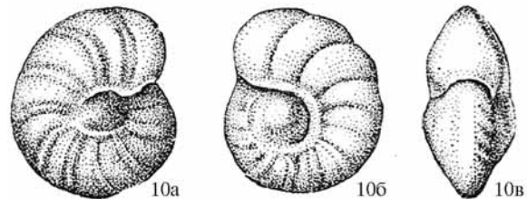
Cibicides (Anomalinoides) insignis Lipnik [Липник, 1979; с. 124, т. 46, фиг. 10, а-в]; Днепроовско-Донецкая, Конско-Яльнская и Причерноморская впадины, кампан
