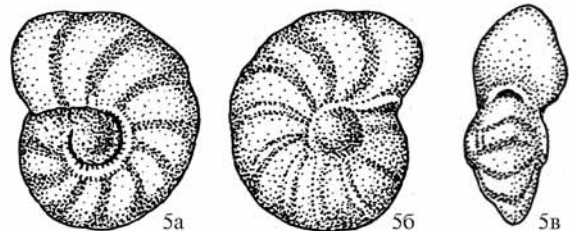
Anomalina insignis (Lipnik) [Горбенко, 1974; с. 45, т. 6, фиг. 4, а-в]; Донбасс, нижний кампан Рис. 7. Вид-индекс Anomalinoides insignis (Lipnik) — форма, легко и однозначно идентифицируемая
