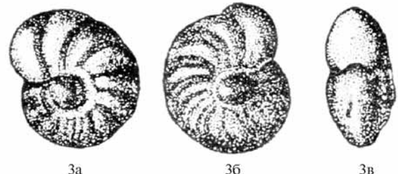
Cibicides (Anomalinoides) insignis Lipnik [Раузер-Черноусова и др., 1963; с. 102, т. XXI, фиг. 3, а-в], Днепроовско-Донецкая впадина, кампан
