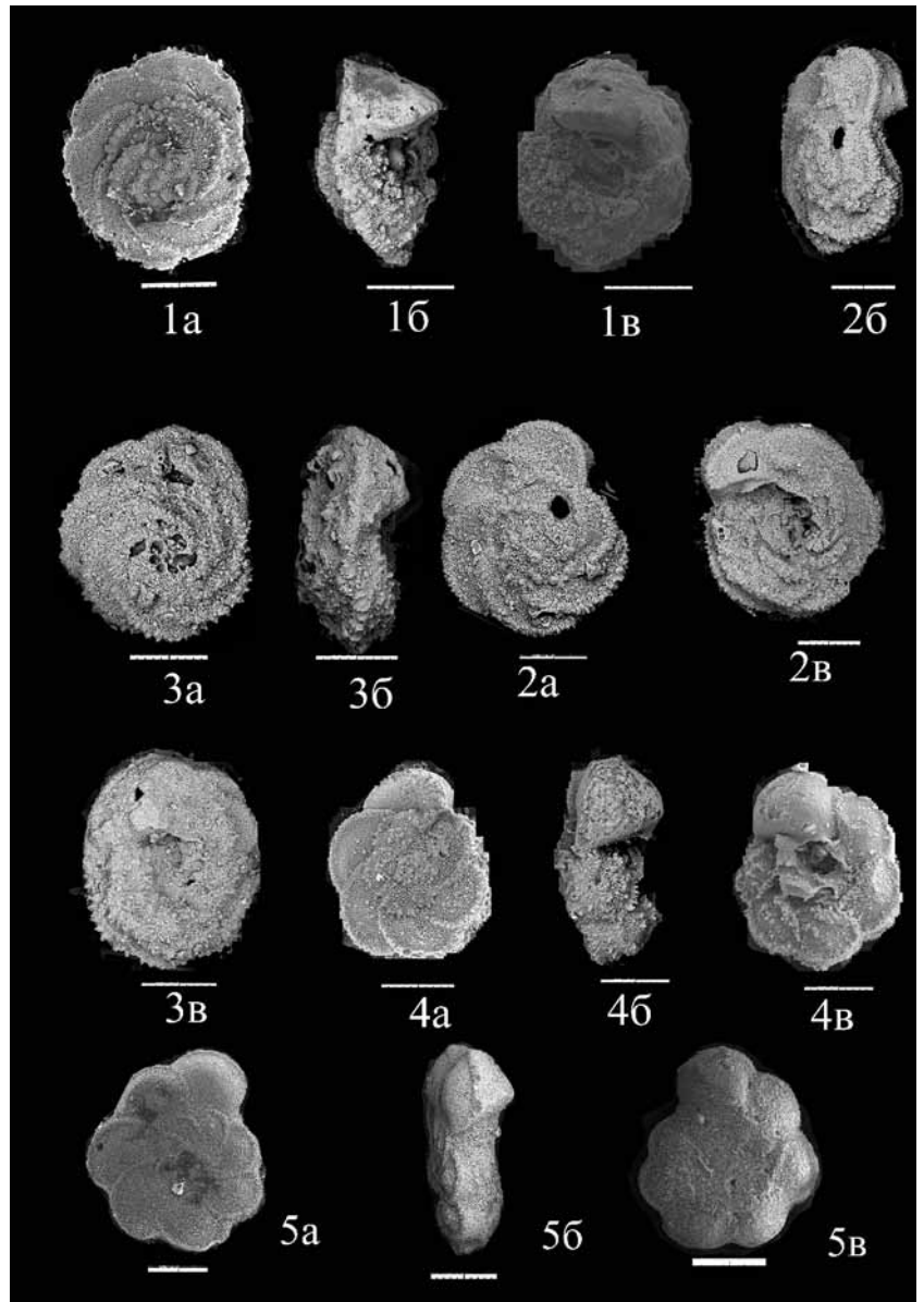
Рис. 9. Планктонные фораминиферы из разреза Алан-Кыр: 1а-в — Globotruncanina elevata (Brotzen), образец 13-2-13, верхняя часть верхнего сантона; 2а-в — Globotruncana arca (Cushman), образец 13-2-15, нижний кампан; 3а-в — Contusotruncana fornicata (Plummer), образец 13-2-12, верхний сантон; 4а-в — Globotruncana bulloides Vogler, образец 13-2-12, верхний сантон; 5а-в — Concavotruncana concavata (Brotzen), образец 13-2-12, верхний сантон. Линейка 150µm
