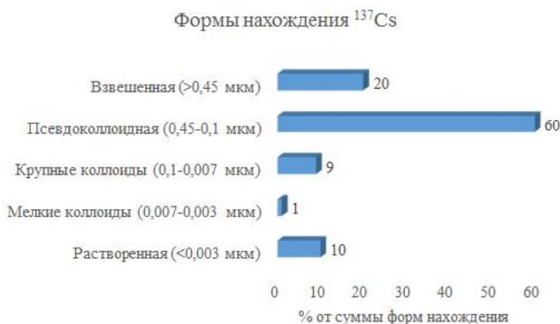
Рис. 2. Формы нахождения ^{137}\text{Cs} в модельных растворах / Fig. 2. Speciation of ^{137}\text{Cs} in water in laboratory scale experiments
