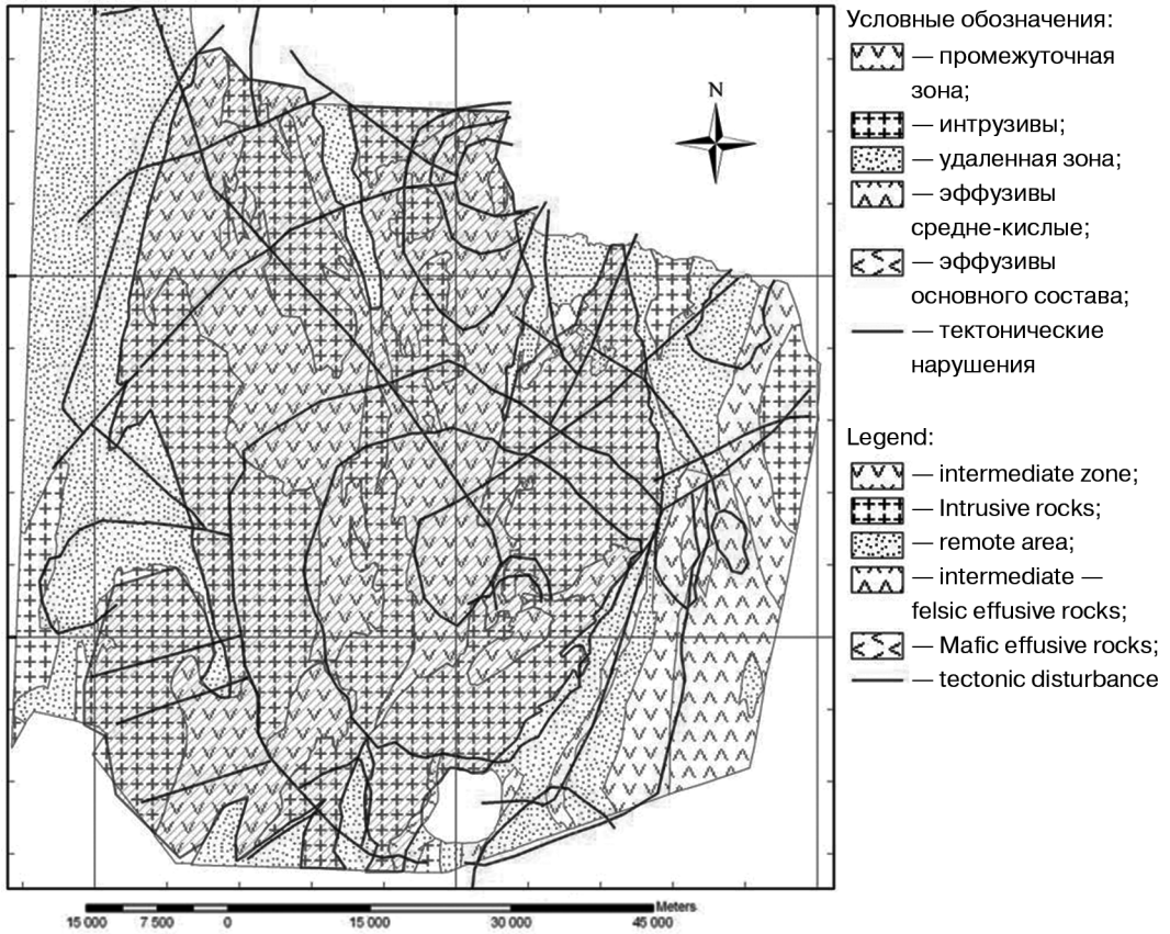
Рис. Карта-схема тектонических нарушений Восточного Оренбуржья [Fig. A schematic map of tectonic disturbances of the East Orenburg region]
