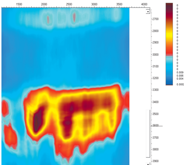
Fig. 17. VPRTM: Impedance
