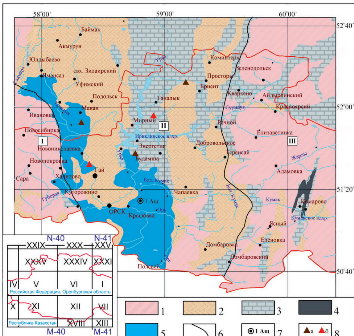
Рис. 1. Оренбургский сегмент Магнитогорского прогиба и сопредельные площади. Геологические формации, слагающие верхнюю часть разреза
