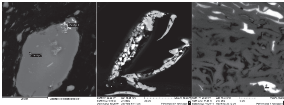
Рис. 7. Рутил в угольном веществе: 1 – рутил (спектр 1) в кварцевом зерне (спектр 2); 2 – рутил (ярко-белое) в угольных порах; 3 – рутил (белое) в инертините. Тунгусский бассейн, р. Горбиачин, контактовый антрацит.
