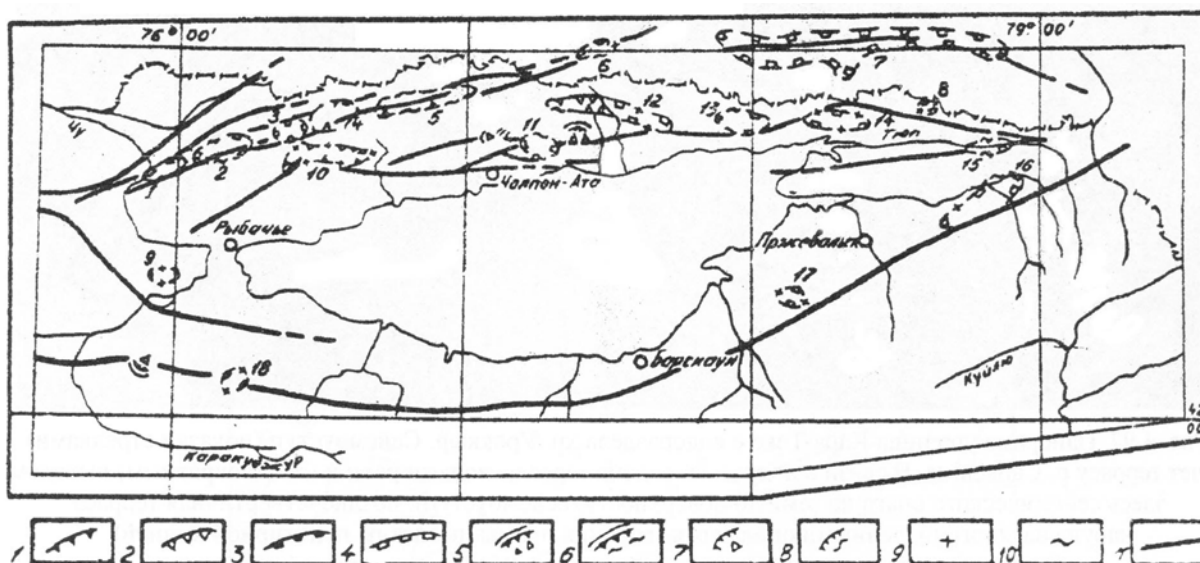
Рис. 4. Карта сейсмодислокаций Иссык-Кульской впадины и её горного обрамления [10].
