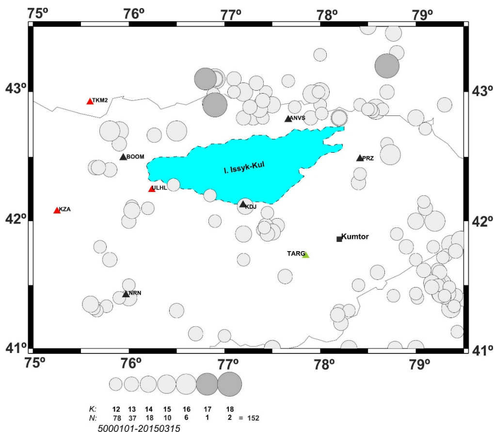
Рис. 2. Карта эпицентров землетрясений K=12-18 на территории Иссык-Кульского региона за историческое и современное время (составила С. Молдобекова).
