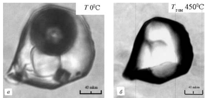
Рис. 3. Изменение включений в процессе термометрических исследований в кварцах Верхне-Шибановского месторождения: a — при 0^{\circ}\text{C} , б — при 450^{\circ}\text{C}
