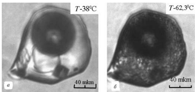
Рис. 2. Изменение включений в процессе криометрических исследований в кварцах Верхне-Шибановского месторождения: a — при -38^{\circ}\text{C} , б — при -62,3^{\circ}\text{C}
