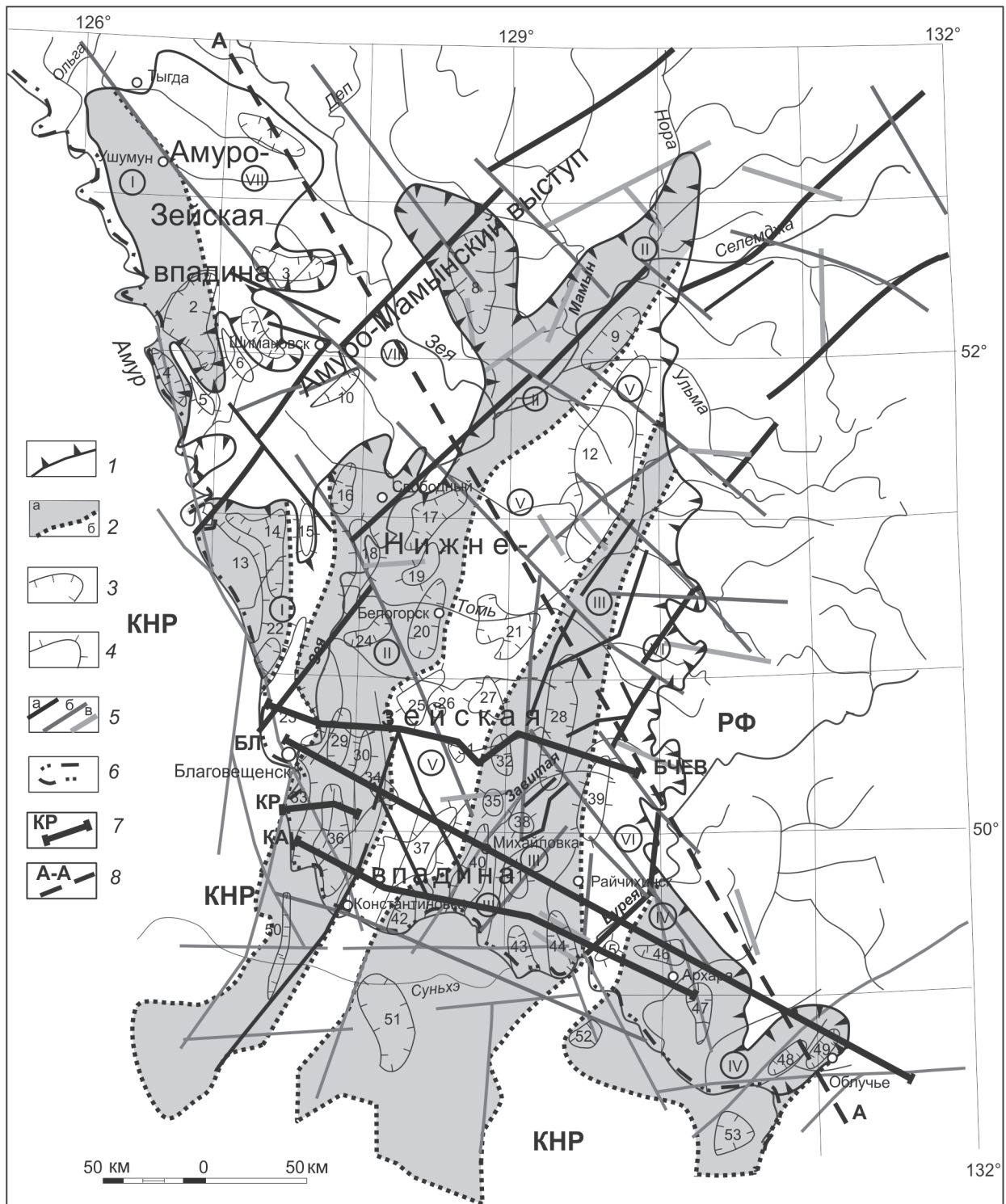
Рис. 1. Тектоническая схема Зейско-Буреинского бассейна [25, 27].
