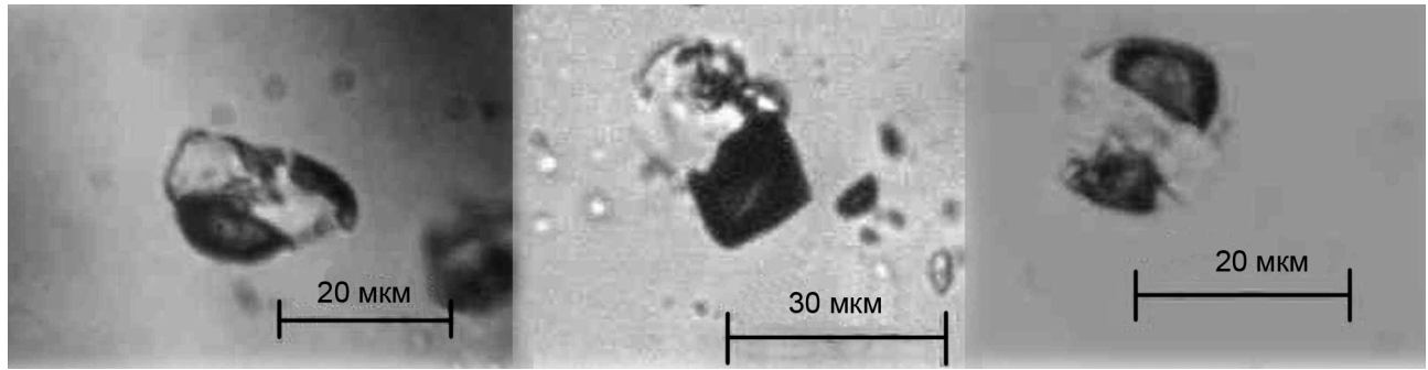
Рис. 6. Расплавные включения в порообразующем кварце гранитов Дальнегорского боросиликатного месторождения.
