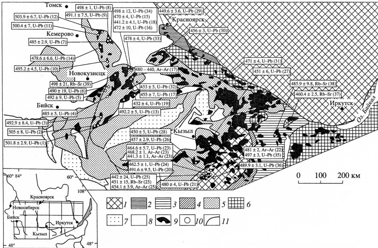
Рис. 1. Схема расположения раннепалеозойских гранитоидных батолитов Алтае-Саянской складчатой области. 1 – Сибирский кратон; 2 – рифтогенные комплексы ( R_3 ); 3–5 – островодужные комплексы (3 – позднерифейские, 4 – вендские, 5 – кембрийские); 6 – террейны с раннекаледонской ремобилизацией коры; 7 – орогенные молассы и осадочные бассейны (поздний кембрий–силур); 8 – геологические комплексы среднего палеозоя–раннего мезозоя; 9 – гранитоидные батолиты; 10 – точки геохронологического опробования гранитоидов и габброидов, в рамках вынесены: возраст (млн. лет), метод изотопного датирования и номер массива (в скобках); 11 – основные разломы. Цифрами в скобках обозначены массивы, для которых проведены изотопно-геохронологические исследования: 1 – Садринский, 2 – Базлинский, 3 – Верхнекондомский, 4 – Колосовский, 5 – Тебинский, 6 – Лужбинский, 7 – Малодудетский, 8 – Кайдаловский, 9 – Карнаольский, 10 – Ударнинский, 11 – Кожуховский, 12 – Краснокаменский, 13 – Аскизский, 14 – Центральнинский, 15 – Туимо-Карышский, 16 – Белоюсский, 17 – Сайгачинский и мелкие штоки Сорского рудного поля, 18 – Туимо-Карышский, 19 – Саксырский (Сырский), 20 – Эрзинский, 21 – Тесхемский, 22 – Нижнеулорский, 23 – Башкымугурский, 24 – Матутский, 25 – Кокмолгаргинский, 26 – Шурмакский, 27 – Каахемский, 28 – Бренский, 29 – Шумихинский, 30 – Бельковский, 31 – Катунский, 32 – Чалпанский, 33 – Юлинский, 34 – Туимо-Карышский, 35 – Баянкольский, 36 – Чжаргалантский, 37 – Ихе-Хайгасский, 38 – Гадрусский, 39 – Солгонский.
