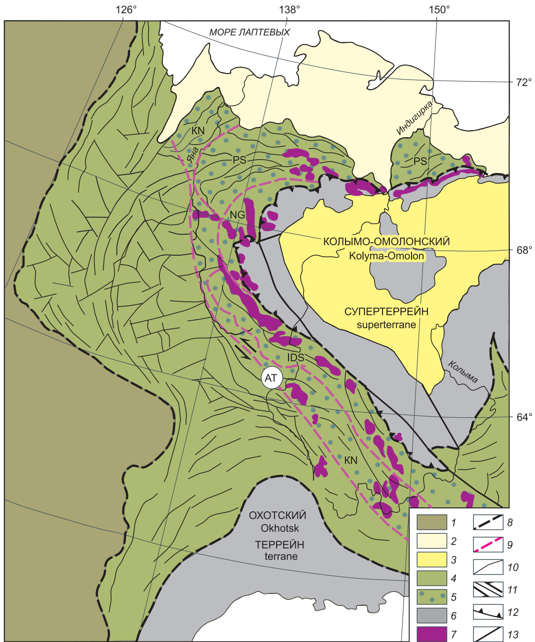
Рис. 1. Тектоническая схема Верхояно-Колымской складчатой системы.
