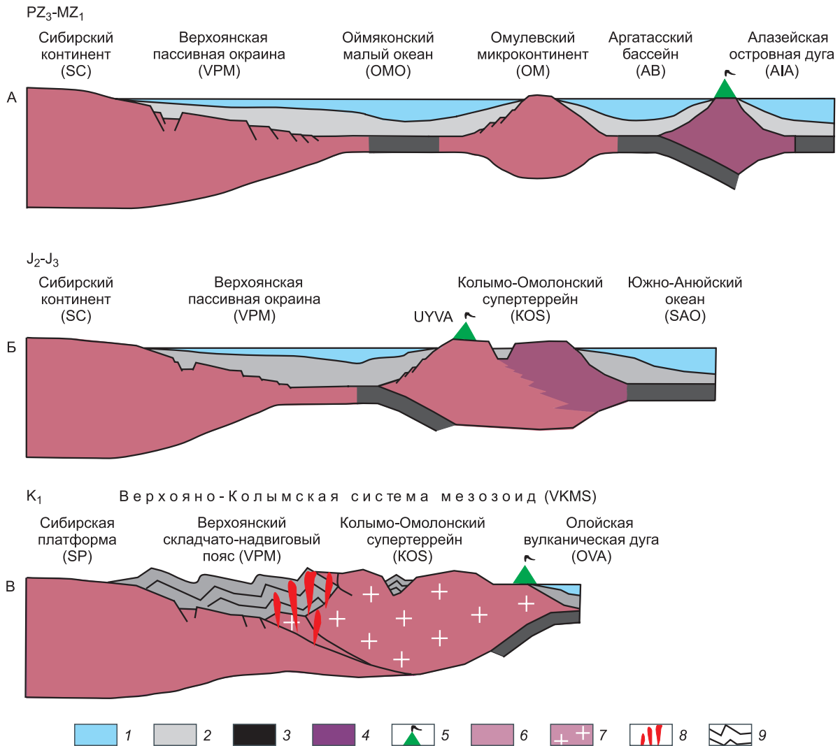
Рис. 2. Схема тектонического развития Верхояно-Колымской системы мезозойд.
