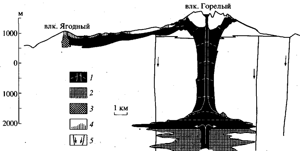
Рис. 7. Предполагаемое строение магмопитающей системы вулкана Горелый и схема развития его последнего эффузивного извержения (разрез в плоскости питающей его дайки): 1 - магма в очаге, в дайке и потоках, контуры канала в плоскости дайки и граница раздела магмы андезитового (вверху) и андезитобазальтового (внизу) состава; 2 - породы краевых групп и кумулаты; 3 - жерловина вулкана Ягодный; 4 - плоскости трещин; 5 - кальдерные сбросы. Пояснения см. в тексте.
