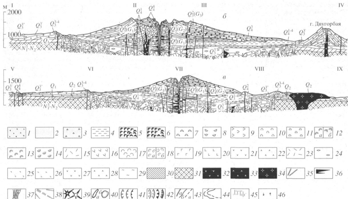
Рис. 2. Геологическая карта вулкана Горелый (а) и разрезы по линиям I–IV (б) и V–IX (в). Современные и нерасчлененные позднплейстоцен-голоценовые отложения: 1 – пеплы, глыбы и шлаки последних извержений вулкана; 2 – аллювий; 3 – отложения обвалов, селей, лахаров; 4 – комплекс водно-ледниковых, аллювиально-пролювиальных и озерных отложений с прослоями вулканических пеплов и шлаков ( Q_3^4 - Q_4^4 ). Поздний голоцен ( Q_4^4 , 2,6 тыс. лет назад – ныне); 5, 6 – соответственно андезитобазальты и андезиты последней серии эффузивных извержений вулкана (XVIII в.). Средний голоцен ( Q_4^3 , 5,0–2,6 тыс. лет назад): 7 – андезитобазальты; 8 – андезиты. Ранний голоцен ( Q_4^2 , 8,0–5,0 тыс. лет назад): 9 – базальты; 10 – андезитобазальты; 11 – андезиты. Древний голоцен ( Q_4^1 , 11,0–8,0 тыс. лет назад): 12 – лавы (а) и шлаки (б) базальтов; 13 – андезитобазальты; 14 – андезиты. Верхи позднего плейстоцена ( Q_3^4 ): 15 – пемзы и пемзовые туфы вершинной кальдеры вулкана Мутновский-III ( M_3^2 ); 16 – базальты; 17 – андезитобазальты; 18 – андезитовые лавы (а) и агломераты-агглютинаты (б). Поздний плейстоцен ( Q_3^{3-4} ), комплекс ранне-посткальдерных моногенных вулканических аппаратов и продуктов их деятельности: 19 – базальты; 20 – андезитобазальты; 21 – андезиты; 22 – дациты. Поздний плейстоцен ( Q_3^3 ): 23 – дацитовые пемзы заключительного этапа кальдероформирующих извержений ( Q_3^3 ); 24 – дацитовые, андезиодацитовые и андезитовые пемзы и игнимбриты главного периода кальдерообразующих извержений Гореловского центра ( Q_3^3 ). Средний плейстоцен ( Q_2 ), породы докальдерного комплекса пра-Горелого и соседних вулканов: 25 – базальты; 26 – андезитобазальты; 27 – андезиты; 28 – дациты. Ранний-средний плейстоцен ( Q_{1-2} ): 29 – дацитовые игнимбриты (на разрезе I–IV). Ранний плейстоцен ( Q_1 ): 30 – лавовые покровы (базальты – андезитобазальты) и останцы стратовулканов (базальты – андезиты). Поздний миоцен – плиоцен ( N_1^2 - N_2 ): 31 – слабодислоцированная толща контрастных, базальтоидных и кислых вулканитов с экструзиями биотит-роговообманковых риолитов (алнейская серия). Породы экструзий: 32 – базальты; 33 – дациты; 34 – риолиты; 35 – дайки; 36 – силлы (на разрезах); 37 – эруптивные брекчии жерловин; 38 – останцы древних разрушенных вулканов; 39 – шлаковые конусы, молодые и частично разрушенные ранние; 40 – лавовые блоки (а) и воронки фреатических взрывов (б); 41 – гребни кратеров (от древних к молодым); 42 – гребни и бровки кальдерных уступов (от ранних к молодым); 43 – разрывные нарушения (а – с установленным смещением, б – безамплитудные, в – затухающие и погребенные); 44 – геологические границы между возрастными комплексами и отдельными телами (внутриформационные); 45 – зоны измененных пород; 46 – термальные источники и паргазовые струи. Членение голоцена – в соответствии с климатической периодизацией и ^{14}C -датировками границ [26].
