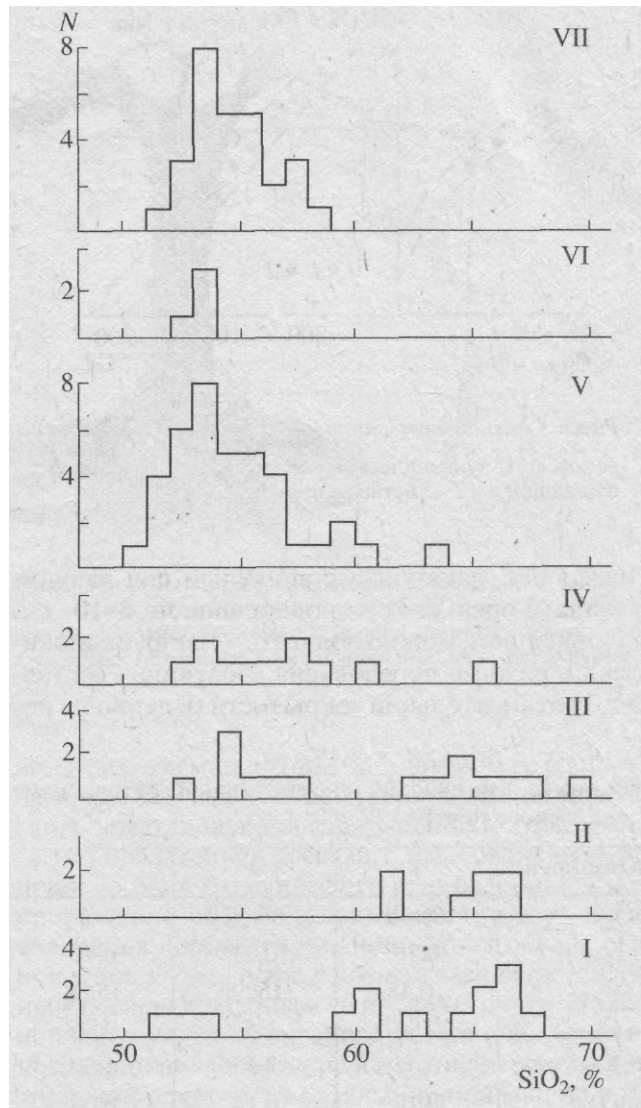
Рис. 5. Распределение составов пород в возрастных комплексах Гореловского вулканического центра: I—III - докальдерный, синкальдерный и ранний посткальдерный комплексы соответственно; IV - вулкан Горелый-1; V - вулкан Горелый-2; VI - вулкан Горелый-3; VII - вулканы рифтовой системы. На вертикальной оси - число анализов.
