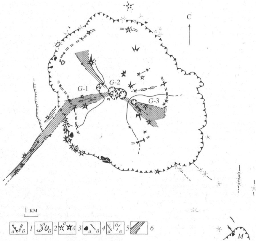
Рис. 4. Структурная схема Гореловского вулканического центра: / - контур кальдеры вулкана Горелый по бровке уступа (а) и очертания блока предполагаемой дополнительной просадки, маркируемые ансамблем эксцентричных прорывов (б); 2 - кратеры (я) и лавовые бокки (б); 3 - шлаковые конусы прорывов докальдерного и ранне-посткальдерного комплексов (а), побочных прорывов вулкана Горелый (б); 4 - экструзии (я) и дайки (б); 5 - разломы с выраженным смещением блоков (я), безамплитудные (б), погребенные и предполагаемые (*); 6 - рифтовая система вулкана; G-1 - G-3 - конусы вулкана Горелый; М - вулкан Мутновский.
