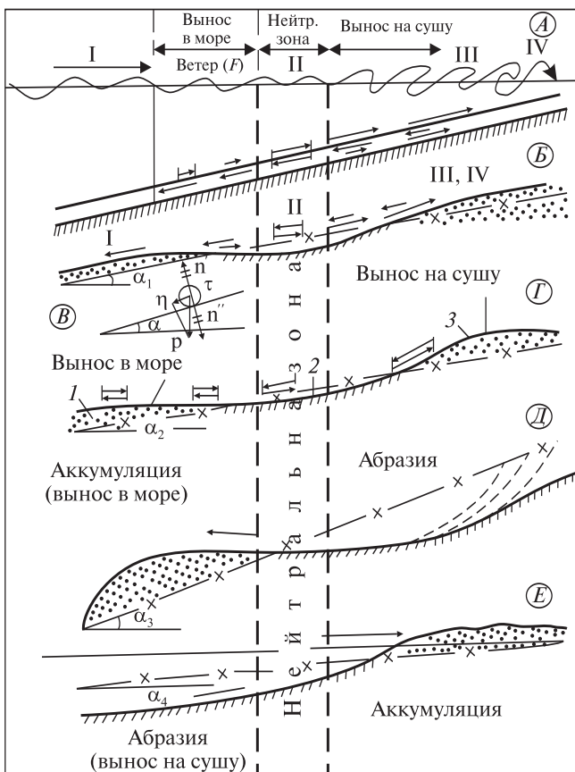
Рис. 2. Условия формирования профиля динамического равновесия [7]
