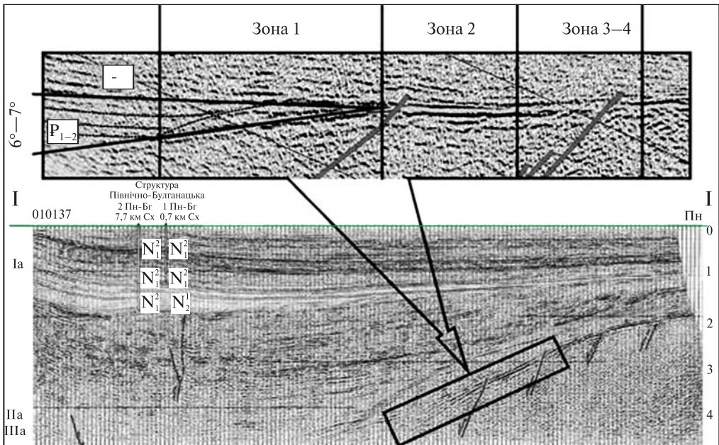
Рис. 4. Зоны профиля динамического равновесия на сейсмическом разрезе I—I
