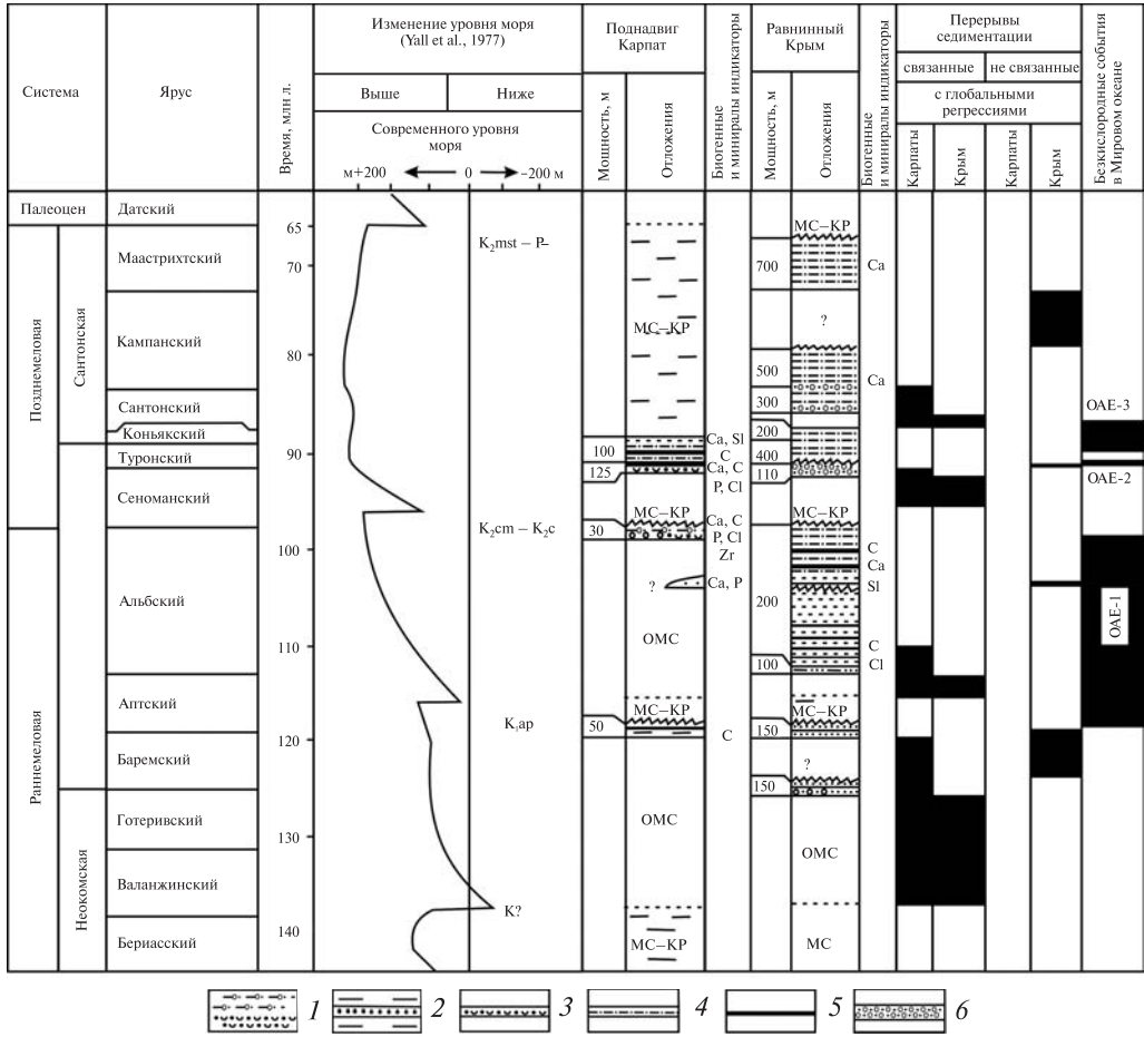
Рис. 1. Седиментологическая летопись палеошельфа Карпато-Черноморского региона. Меловой период: 1 — пески эхинодерматовые и кремнегубковые с глауконитом, спонголиты, гезы, опоки; 2 — кварцевые пески, алевриты; 3 — пески из ракушечного детрита с глауконитом; 4 — нанопланктонные и глинистые илы; 5 — «черные сланцы»; 6 — вулканокластические осадки; ОМС — отсутствие морской седиментации; КР — континентальный режим с денудацией; МС — возможная морская седиментация; ОАЕ — бескислородные события в Мировом океане [9]
