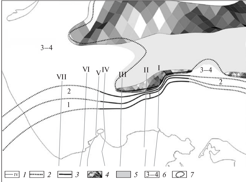
Рис. 3. Схематическая карта распространения геоморфологически обусловленных седиментационных зон палеоцен-эоценового морского бассейна: 1 — линии сейсмических профилей; 2 — предполагаемая граница седиментационной зоны; 3 — фактическая граница седиментационной зоны; 4 — морфоскульптурные возвышения Скифской плиты (на севере — Азовский вал, на юге — Кировско-Тимашевская ступень); 5 — Центральноазовская мульда; 6 — седиментационные зоны палеоцен-эоценового морского бассейна; 7 — контур современной береговой линии
