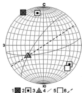
Диаграмма структурных элементов: 1—4 — складка полосчатости: 1 — осевая плоскость; 2, 4 — крылья; 3 — шарнир; 5, 6 — уплощенность энстатита
