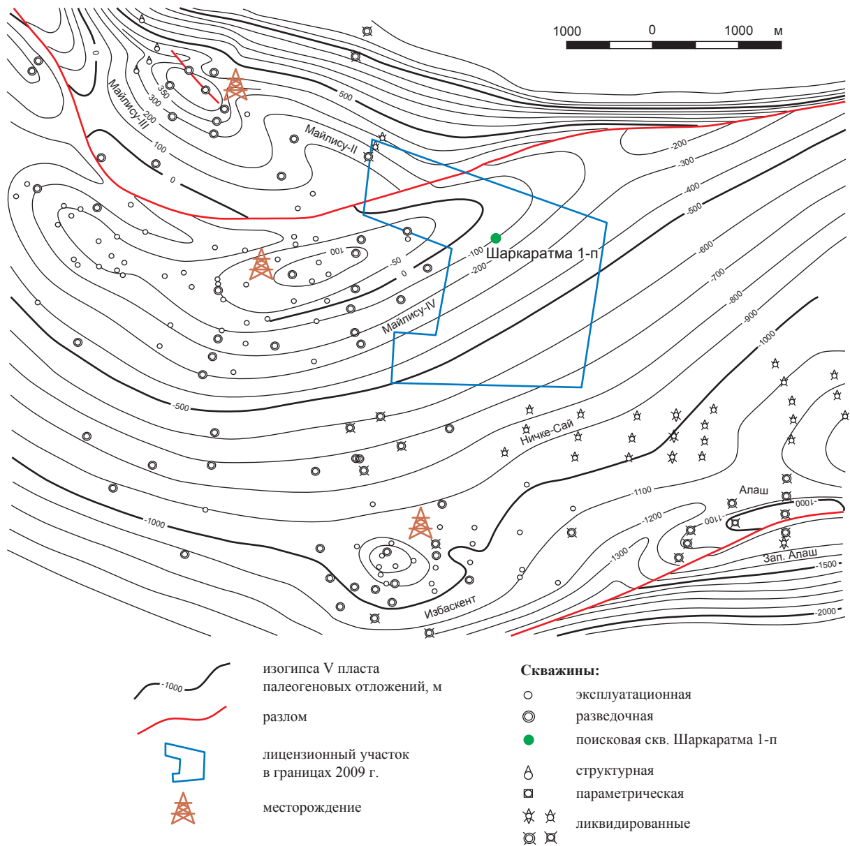
Рис. 3. Майлису-IV выступ: структурная карта по кровле палеогеновых отложений
