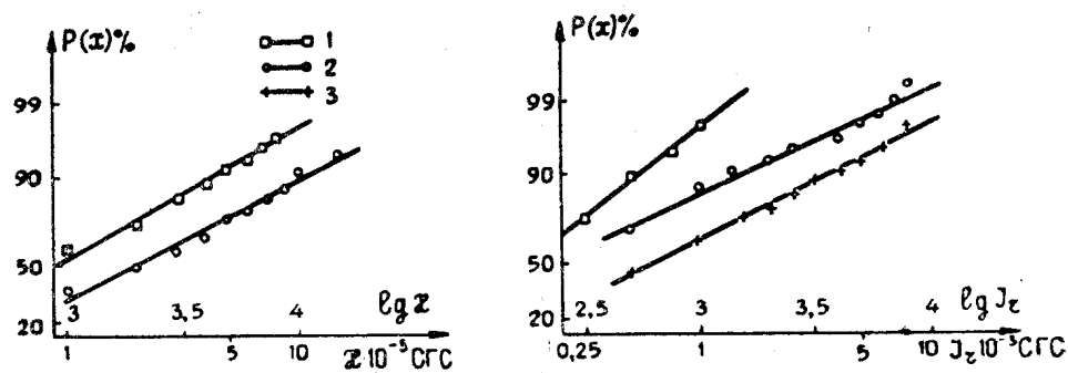
Рис. 2. Графики накопленных частностей для магнитных свойств горных пород Мурюк-Суразовской аномальной зоны. 1 — альбитофиры, 2 — порфиристы, 3 — роговики
