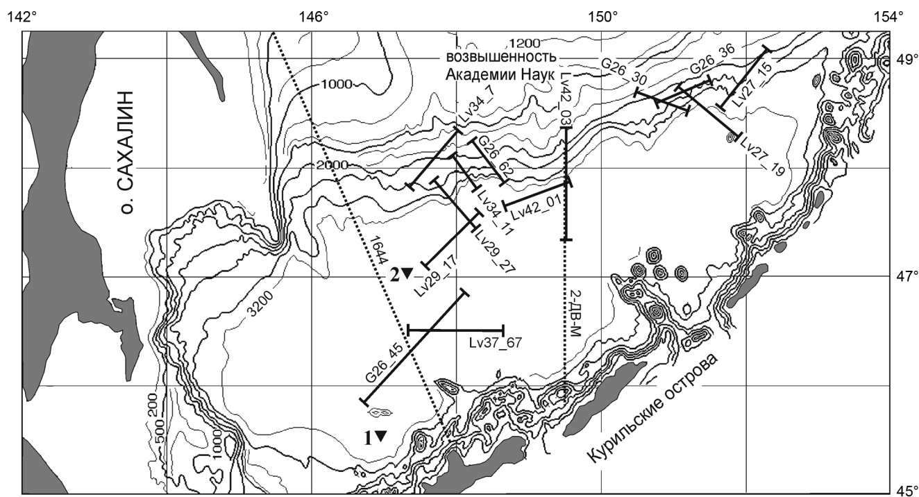
Рис. 1. Расположение профилей НСП (сплошные линии) и ОГТ (пунктирные линии). Залитые треугольники – положение центров профилей №1 и №2 МОВ РБ. Батиметрическая карта составлена А.С. Сваричевским.
