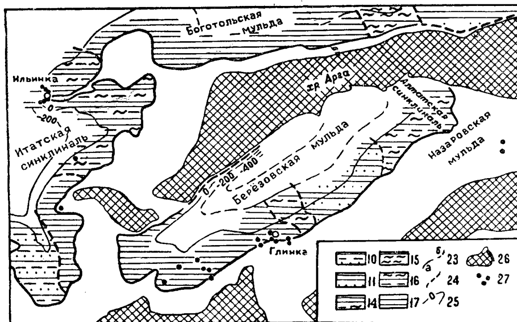
Рис. 3. Литолого-фациальная схема отложений периода формирования Итатского (Березовского) пласта (условные обозначения см. к рис. 2).
