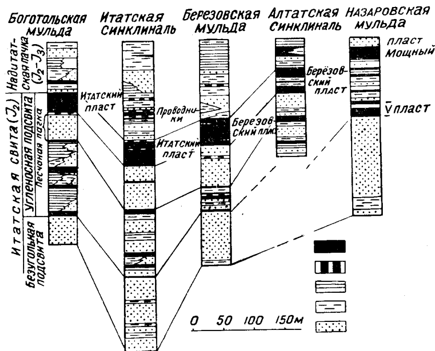
Рис. 1. Схема сопоставления разрезов средней и верхней юры: 1 — угли, 2 — углистые породы, 3 — глины, аргиллиты, 4 — алевролиты, алевриты, 5 — пески, песчаники.
