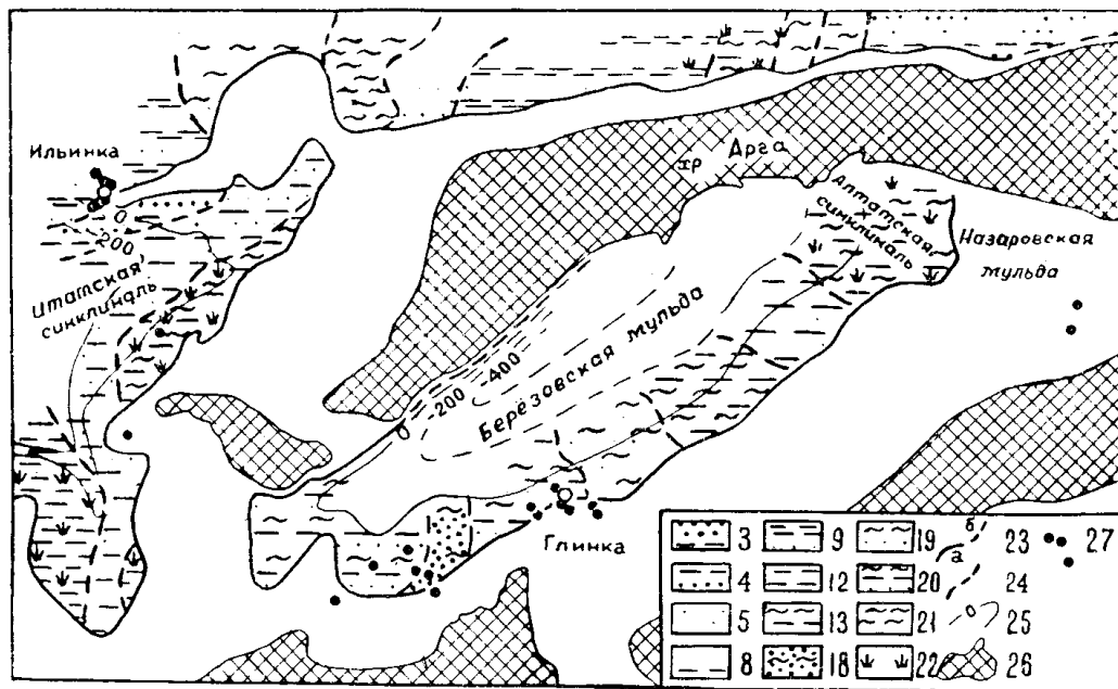
Рис. 4. Литолого-фациальная схема отложений надитатской пачки (условные обозначения см. к рис. 2).
