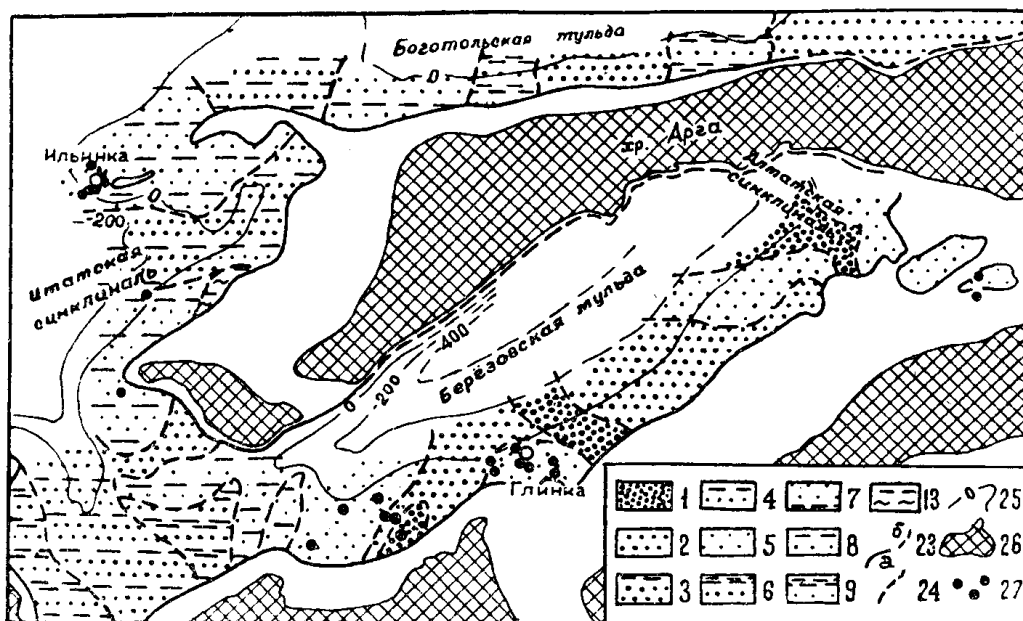
Рис. 2. Литолого-фациальная схема песчаной пачки угленосной подсвиты итатской свиты. Условные обозначения: 1—2—аллювиально-русловые отложения: 1—песчаники крупнозернистые, 2—песчаники среднезернистые; 3—11—руслово-пойменные отложения: 3—песчаники среднезернистые с прослоями алевролитов, 4—песчаники среднезернистые и алевролиты, 5—песчаники мелкозернистые, 6—алевролиты с прослоями среднезернистых песчаников, 7—песчаники мелкозернистые с прослоями алевролитов, 8—песчаники мелкозернистые и алевролиты, 9—алевролиты с прослоями мелкозернистых песчаников, 10—угли, алевролиты, мелкозернистые песчаники, 11—угли с прослоями мелкозернистых песчаников; 12—17—пойменные болотно-озерные и болотные отложения: 12—алевролиты, 13—алевролиты и аргиллиты, 14—угли и алевролиты, 15—аргиллиты с прослоями углей, 16—угли с прослоями аргиллитов и алевролитов, 17—угли; 18—21—дельтаво-озерные и озерные отложения: 18—аргиллиты и крупнозернистые песчаники, 19—аргиллиты и мелкозернистые песчаники, 20—аргиллиты, алевролиты и мелкозернистые песчаники, 21—аргиллиты; 22—наличие в разрезе существенных пропластков угля, 23—граница распространения отложения: а) достоверная, б) предполагаемая; 24—граница литолого-фациальных зон; 25—изогипсы кровли отложений, 26—области развития пород палеозойского фундамента, 27—скважины геохимического опробования.
