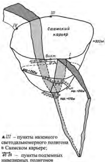
Рис. 1. Общая схема расположения нивелирных и светодальномерных полигонов в районе Саамского разлома (Объединенный Кировский рудник, ОАО «Апатит»)
