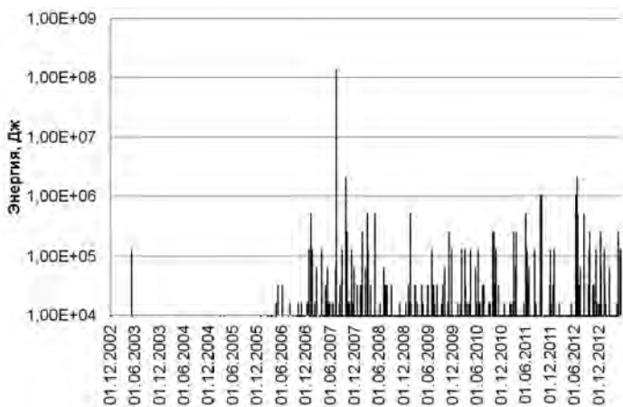
Рис. 3. Сейсмическая активность в районе Саамского разлома ( \pm 200 м от его оси) за 2002–2012 гг.
