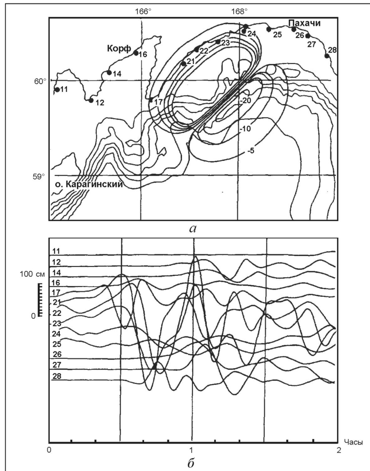
Рис. 5. Остаточные смещения в очаге гипотетического землетрясения в Олюторском заливе (а) и рассчитанные мареграммы для различных пунктов (точки 11–28) побережья (б) [Gusiakov, Marchuk, 1997]
