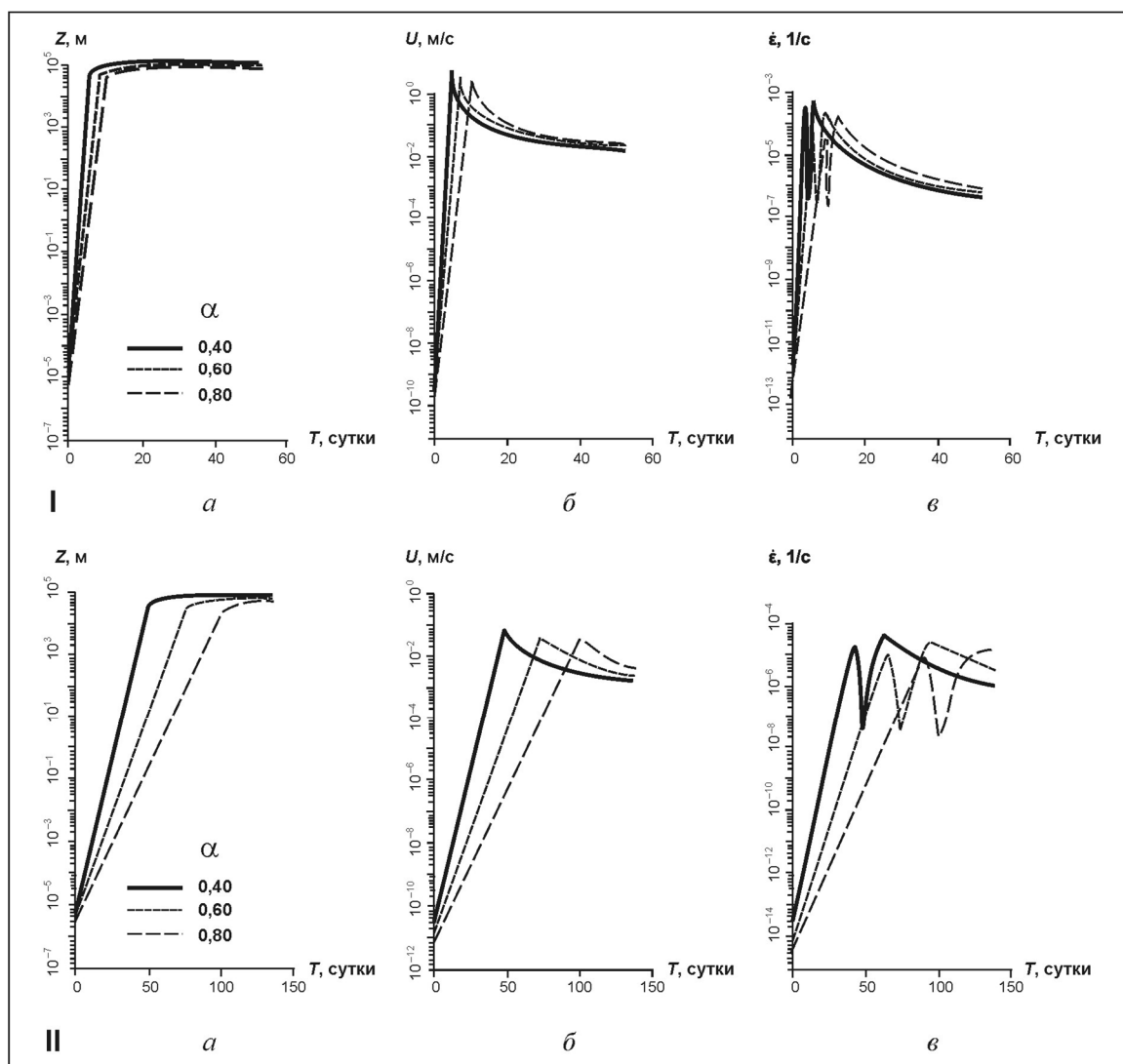
Рис. 1. Зависимость временного изменения расстояния Z , пройденного волной (а), скорости распространения волны U (б) и скорости деформирования \dot{\epsilon} (в) от коэффициентов трения \alpha при \mu = 0,01 (I) и \mu = 0,001 (II)
