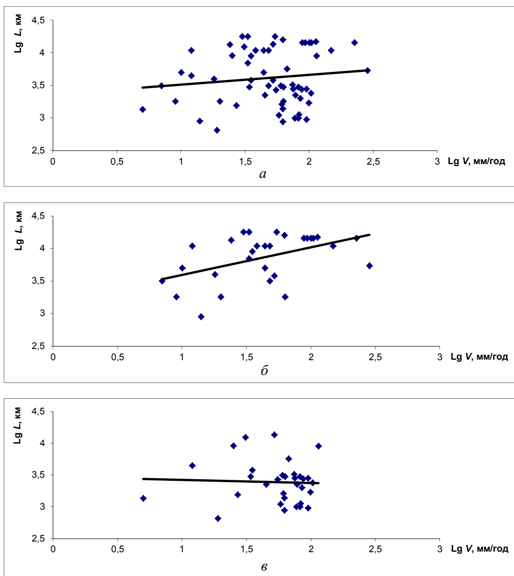
Рис. 5. Данные, характеризующие зависимость Lg L (Lg V) между протяженностями плит L и скоростями их движения по работе [8]:
