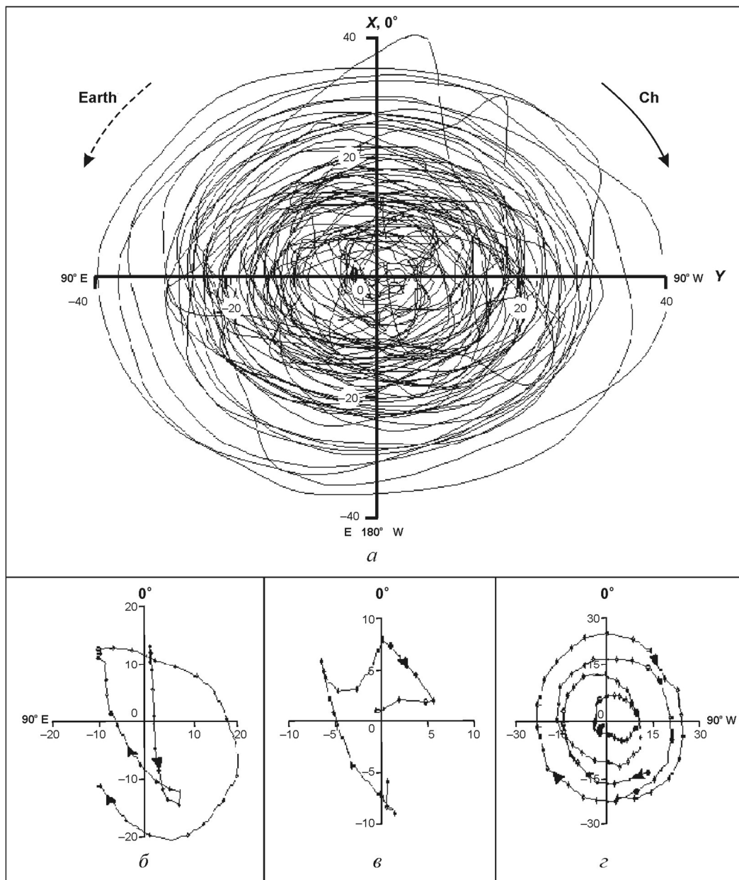
Рис. 1. Траектории нутации полюса планеты, построенные по данным работы [21] в течение 1890–1969 гг. (а) и периодов 1895–1896 гг. (б), 1926 г. (в) и 1960–1964 гг. (г)
