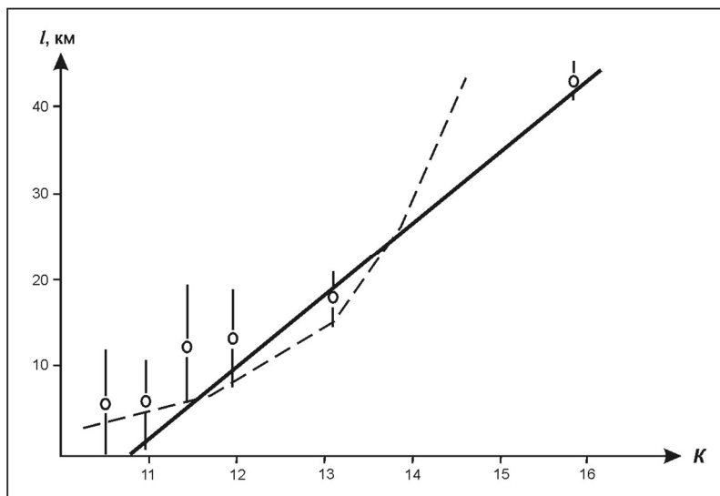
Рис. 5. Зависимость l(K) во всем диапазоне энергетических классов
