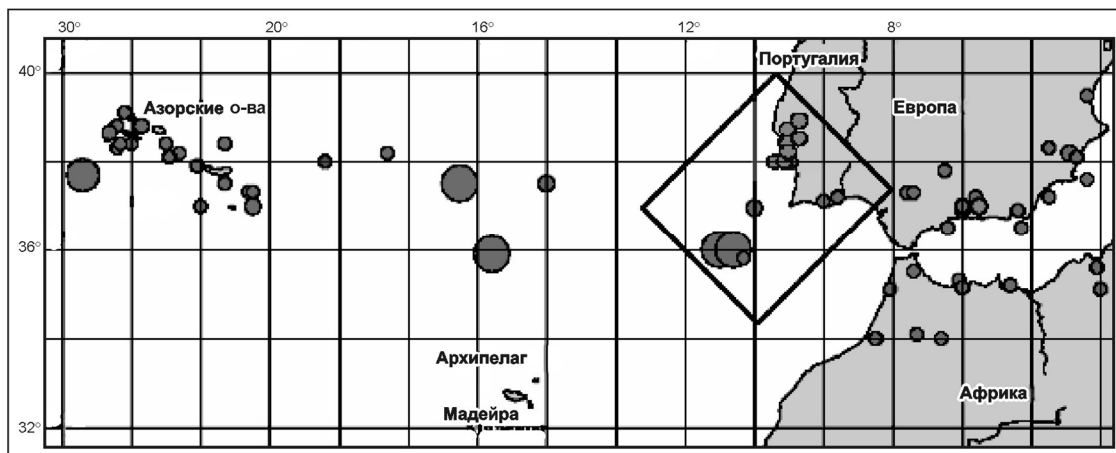
Рис. 2. Сейсмичность западного окончания ( 30^{\circ} W \leq \lambda \leq 0 ) субширотного альпийского тектонического пояса, простирающегося на 160^{\circ} между Тихим и Атлантическим океанами, по данным мирового каталога за 2000 г. до н. э. — 2007 г. [Викулин, Водинчар, Мелекесцев и др., 2007]
