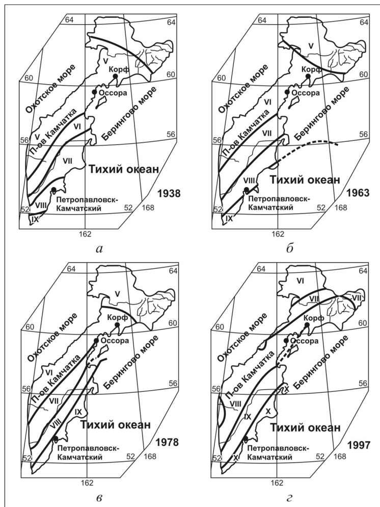
Рис. 2. Карты общего сейсмического районирования Камчатки в 1938 (а), 1963 (б), 1978 (в) и 1997 (з) гг. [Проблемы ..., 2000]
