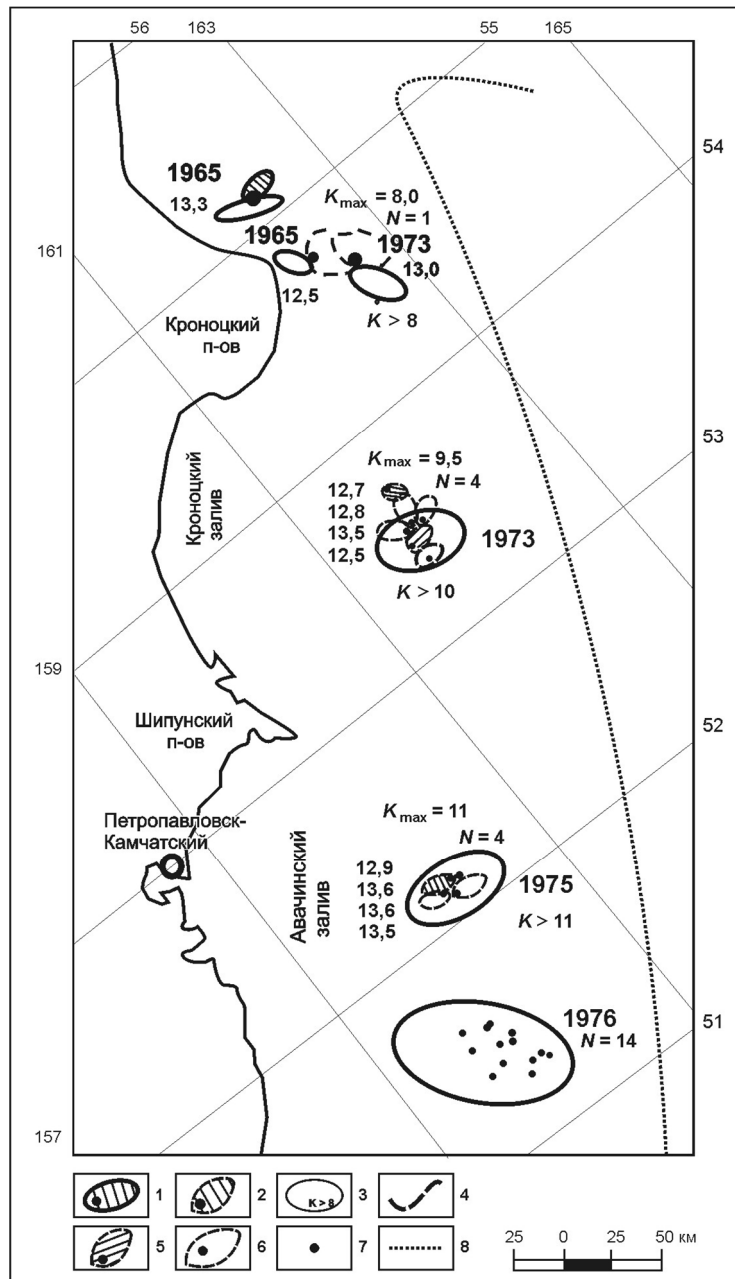
Рис. 4. Зоны молчания и рои:
