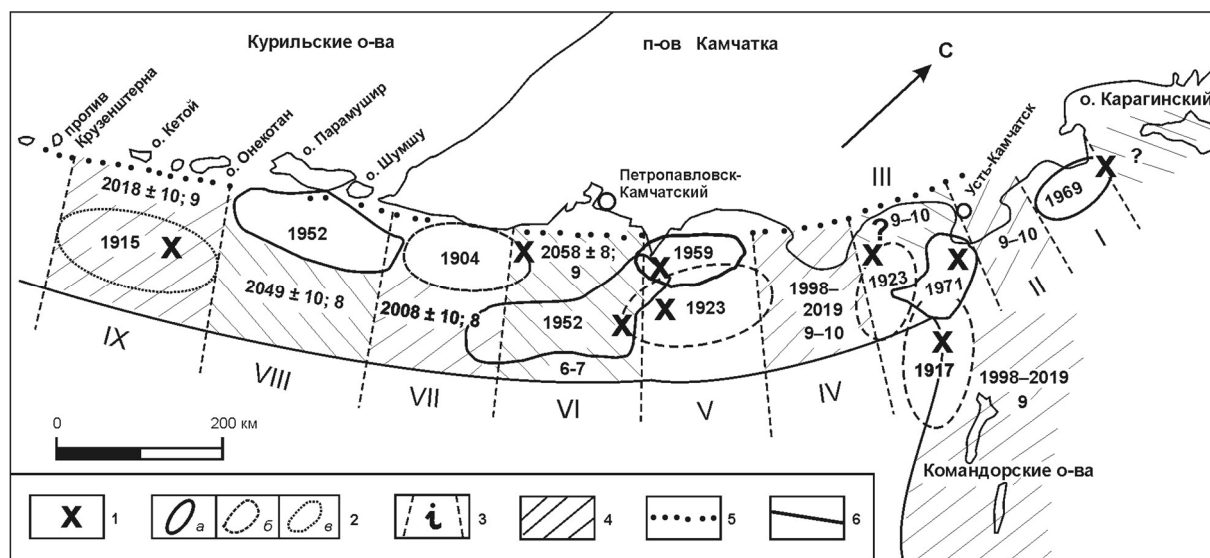
Рис. 3. Прогнозная карта расположения очагов сильнейших камчатских и северо-курильских землетрясений в будущем [6]:
