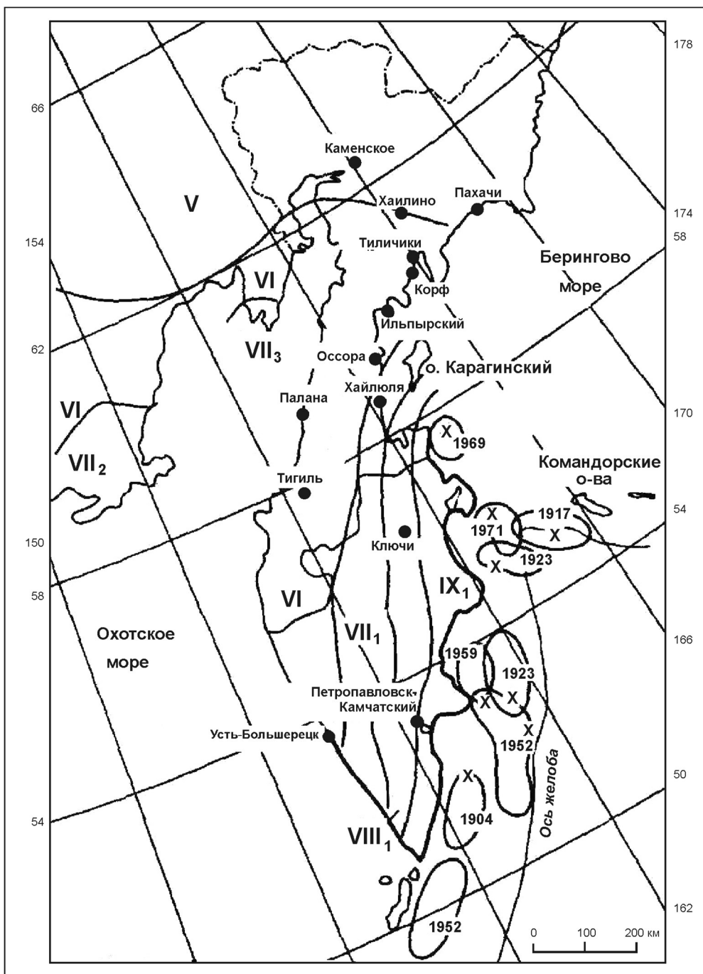
Рис. 1. Карты общего сейсмического районирования ОСР-78 [Сейсмическая..., 1979; СНИП..., 1982] и цунамирайонирования [Соловьев, 1978; Соловьев и др., 1977] Камчатки:
