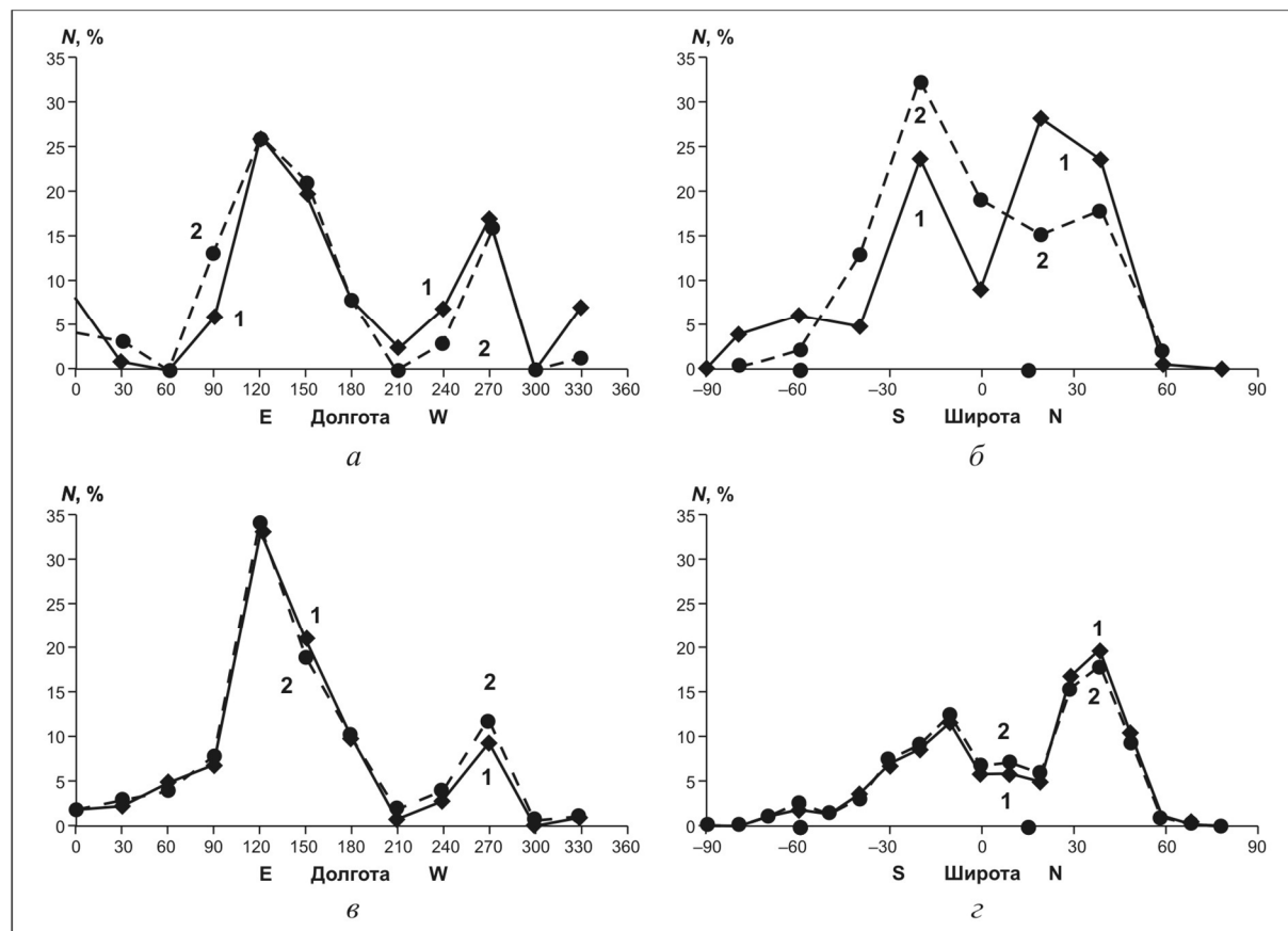
Рис. 5. Долготное (а, в) и широтное (б, з) распределения чисел извержений вулканов (а, б) и гипоцентров землетрясений (в, з) Земли, содержащихся в базе данных [213; 240; Акманова, 2008]:
