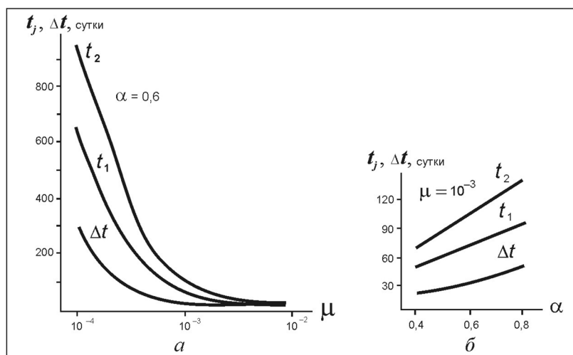
Рис. 5. Зависимость времени максимумов скорости деформирования ( t_1, t_2 ) и временного интервала между ними ( \Delta t ) от коэффициентов неоднородности ( a ) и трения ( b )
