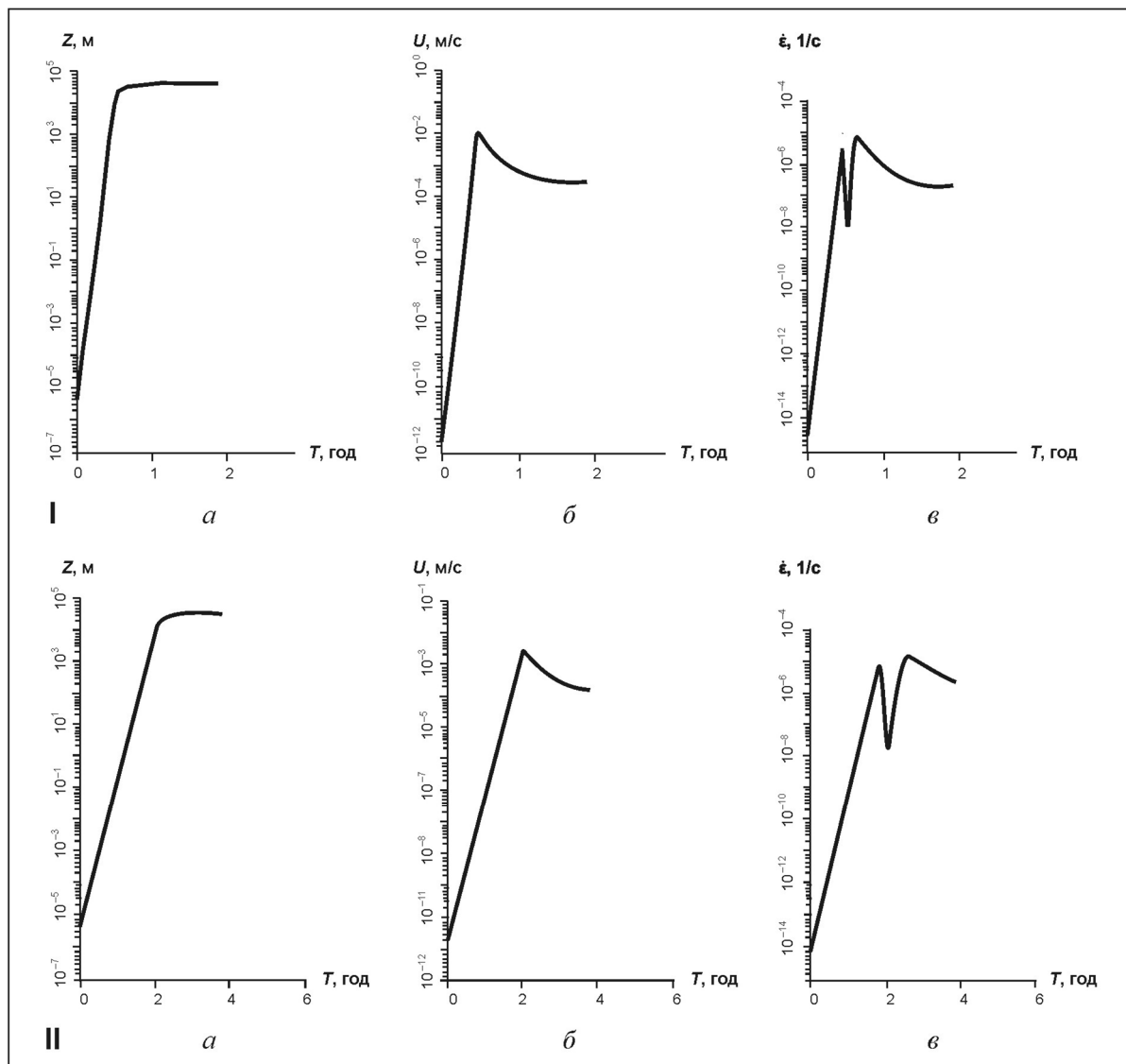
Рис. 2. Зависимость временного изменения расстояния Z , пройденного волной ( a ), скорости распространения волны U ( b ) и скорости деформирования \dot{\epsilon} ( в ) при \alpha = 0,6 , \mu = 0,0005 (I) и \mu = 0,0001 (II)
