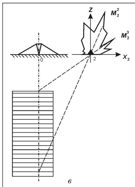
Гистограммы азимутов смещений и геометрические построения для локализации источника вулканического дрожания заключительной стадии Южного прорыва:
