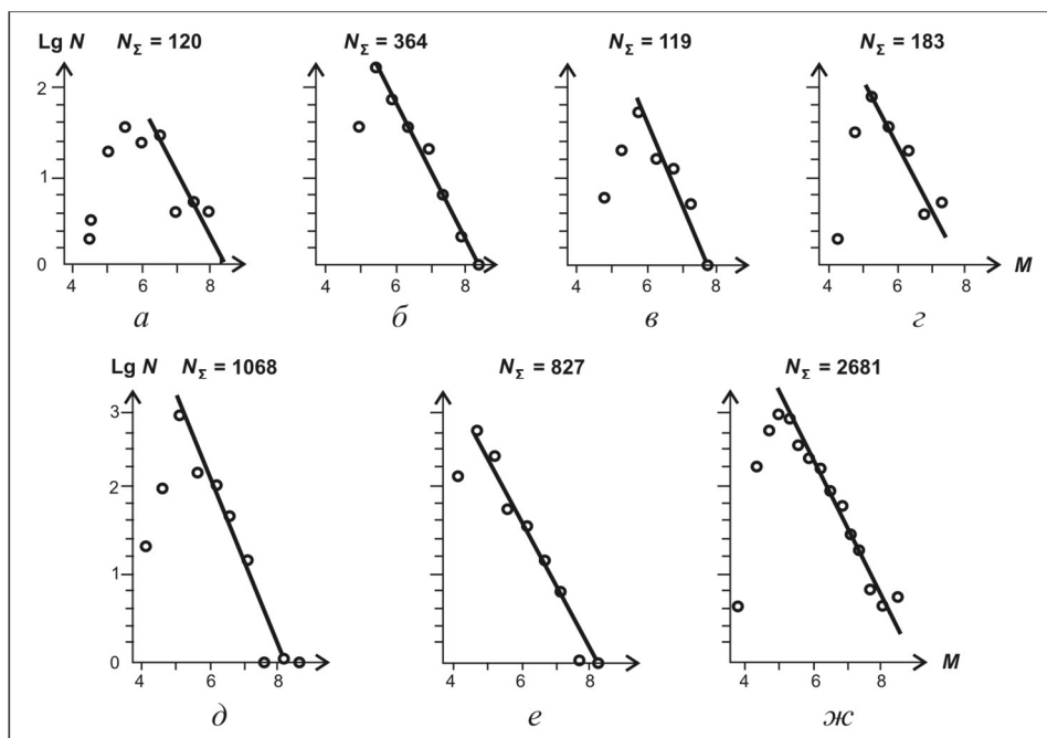
Рис. 4. Графики повторяемости курило-камчатских землетрясений по временным интервалам: 1911–1922 (а), 1923–1937 (б), 1938–1946 (в), 1947–1951 (г), 1952–1957 (д), 1958–1961 (е), 1911–1961 (ж)
