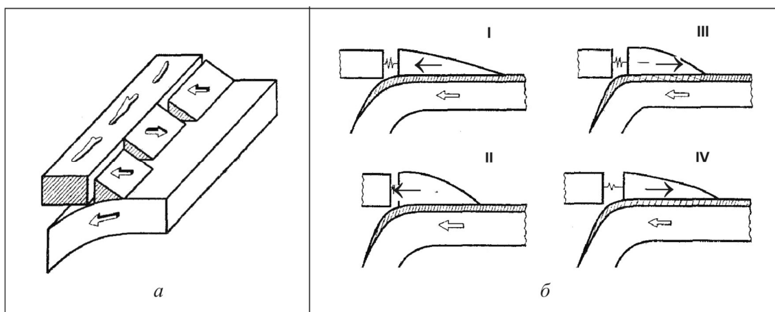
Рис. 3. Блоковое строение фронтального склона островной дуги ( a ) по [9] и стадии сейсмического цикла ( б ) по [10]. Заштрихована контактная зона (см. пояснения в тексте)
