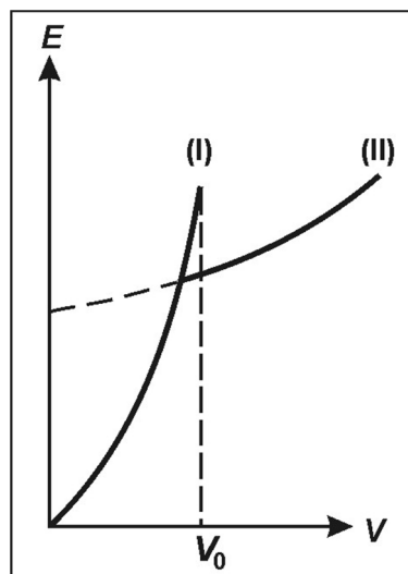
Рис. 3. Волновые решения уравнения СГ:
