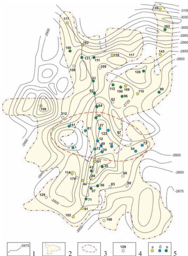
Рис. 2. Схема нахождения нефтей разного типа в пределах залежей пласта Ю 0 Салымского нефтяного месторождения. 1. Изопахиты кровли пласта Ю 0 (ОИГ «Б»); 2. граница зоны, в пределах которой получены притоки нефти из залежей пласта Ю 0 ; 3. зона повышенных пластовых температур; 4. скважина и ее номер; 5. тип нефти: а – тяжелая, б – легкая, в – средняя
