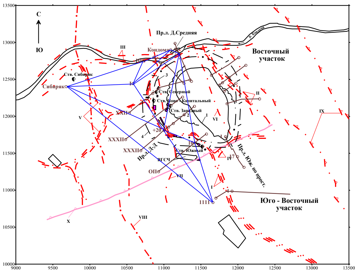
Рис. 1 – Схема структурных блоков Таштагольского месторождения и GPS-полигонов на основе наблюдательной станции на земной поверхности:
