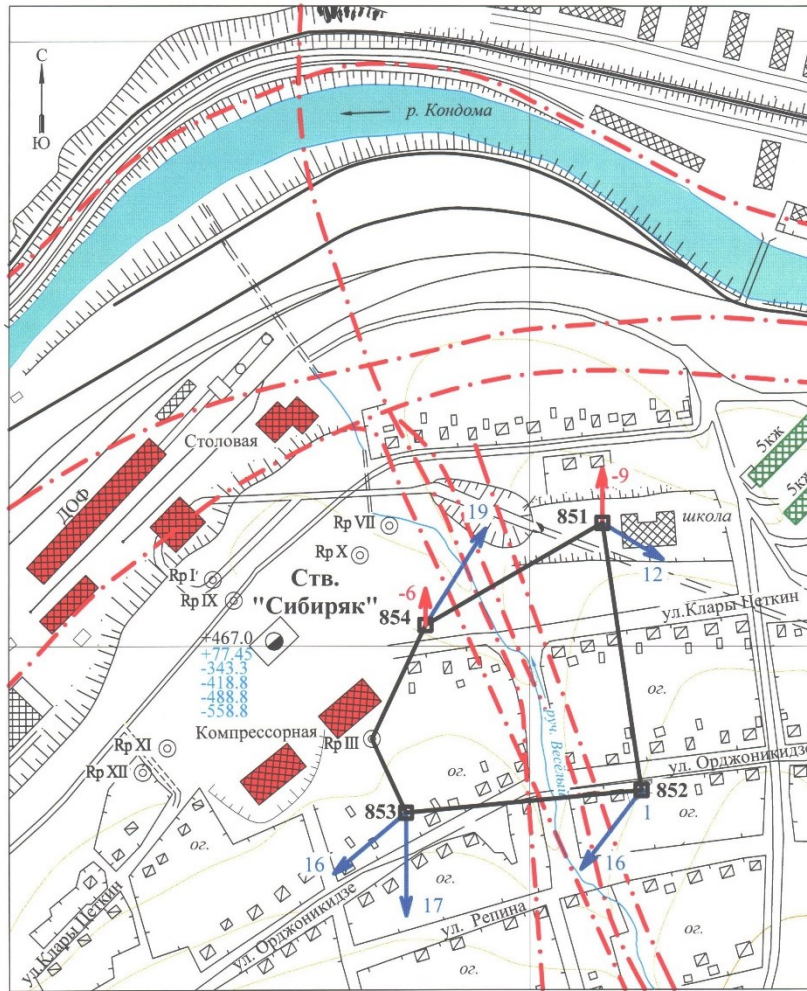
Рис. 3 – Схема геодинамического полигона КузПИ в районе ствола «Сибиряк» и векторы сдвижения за период 1986 – 1987 гг.
