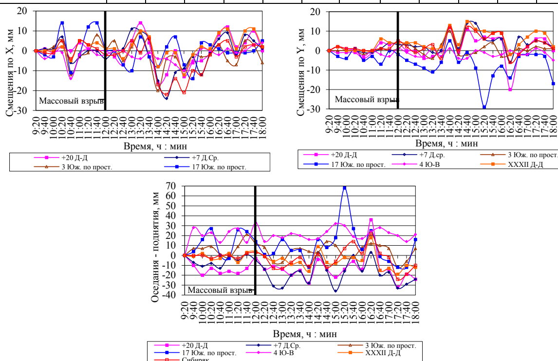
Рис. 5 – Короткопериодные смещения горных пород Таштагольского месторождения, 10.07.2016
