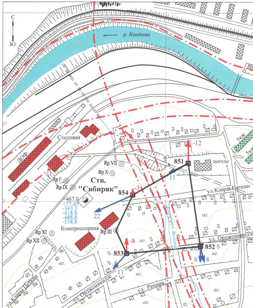
Рис. 2 – Схема геодинамического полигона КузПИ в районе ствола «Сибиряк» и векторы сдвижения за период 1985 – 1986 гг.
