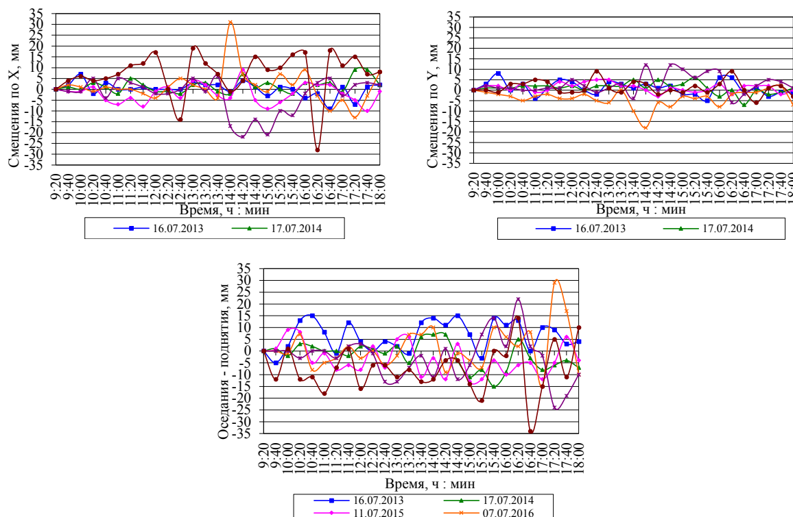
Рис. 4 – Короткопериодные смещения горных пород в районе ствола «Сибиряк» по наблюдениям 2013 – 2017 гг.
