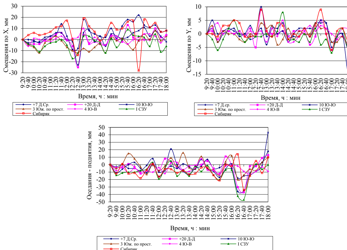
Рис. 6 – Короткопериодные смещения горных пород Таштагольского месторождения, 09.07.2017
