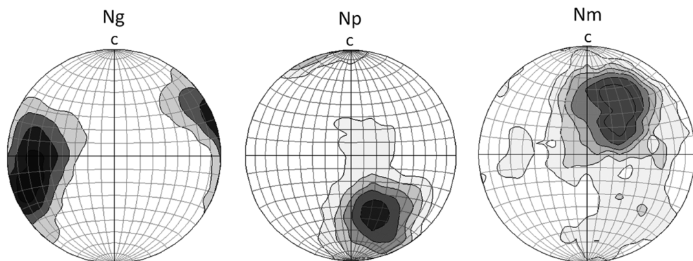
Рис. 2. Генеральная ориентировка осей оптической индикатрисы оливина в пределах детально изученного участка
