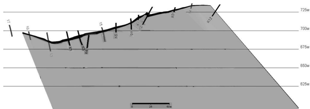
Рис. 5. Склонение рудных тел Южнопогурейского рудопоявления в проекции на вертикальную плоскость, установленное по результатам микроструктурного анализа [ Fig. 5. Dip of ore bodies of Yujinopogureyskoe deposit in projection to the vertical plane based on the results of microstructural analysis]
