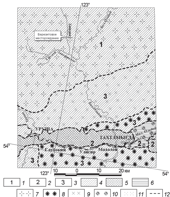
Рис. 2. Ландшафтно-геохимическая карта-схема восточной части Уруша-Ольдойского золотоносного узла
