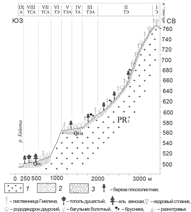
Рис. 3. Ландшафтно-геохимический профиль Березитового месторождения.
