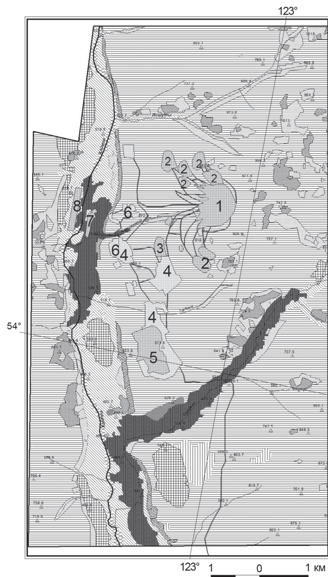
Рис. 4. Ландшафтно-геохимическая карта территории Березитового месторождения и его окрестностей.
