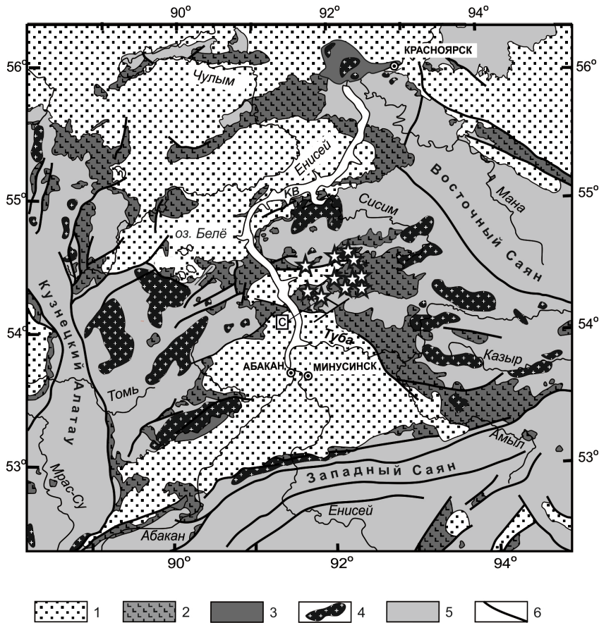
Рис. 1. Схема размещения палеозойских магматических комплексов в северной части Алтае-Саянской складчатой области. Составлена по материалам [Перфилова, Махлаев, Сидорас, 2004; Руднев, 2013]
