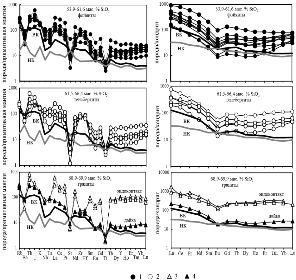
Рис. 5. Графики нормированного распределения элементов в породах Сайбарского массива
