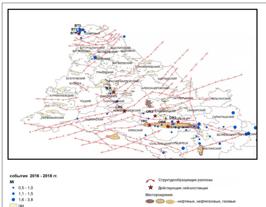
Рис.1 – Регистрация сейсмических событий сетью сейсмических станций «Нефтегаз-сейсмика»
