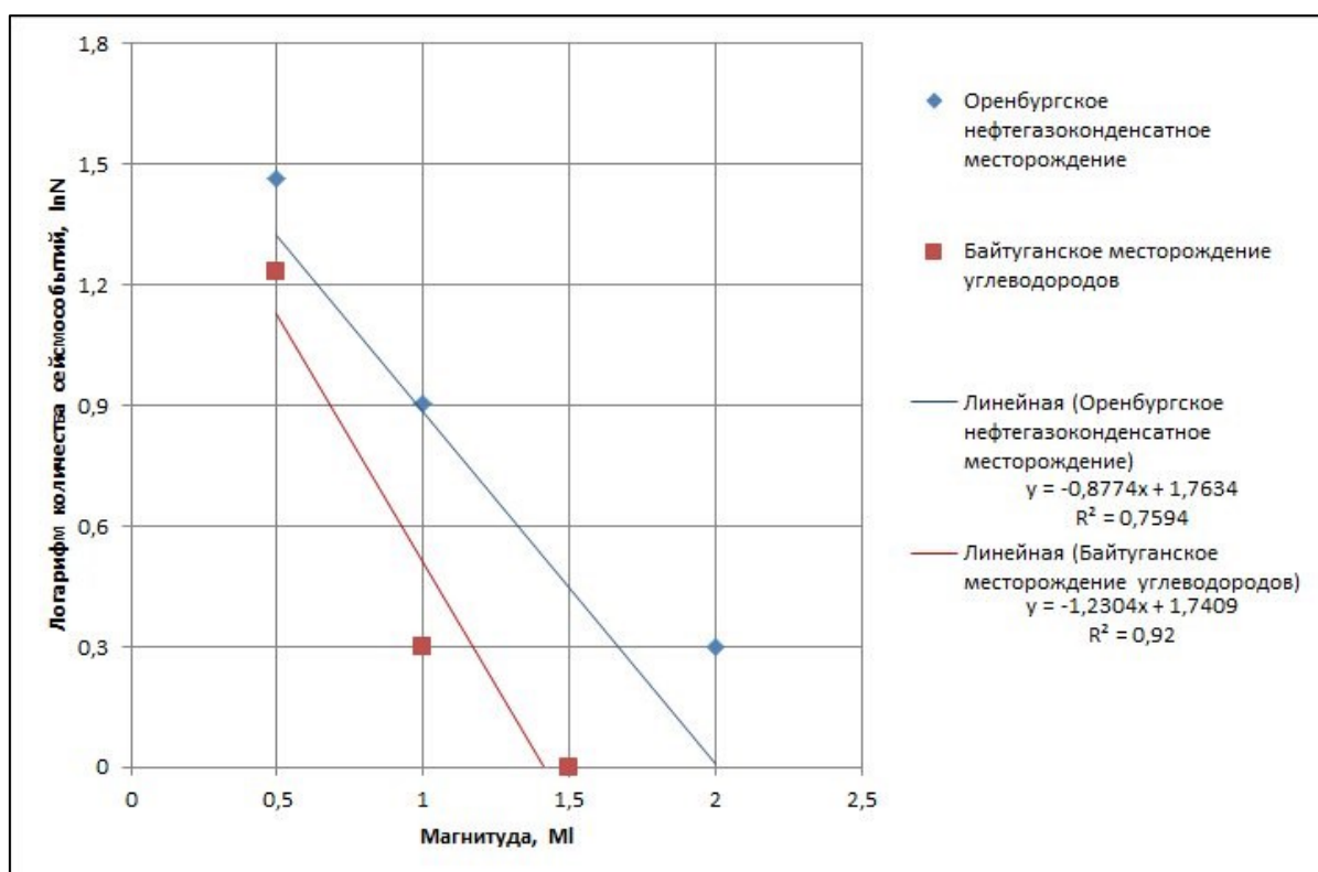
Рис. 2 – График повторяемости сейсмических событий на Оренбургском нефтегазовом месторождении за период 2016 – 2018 гг.
