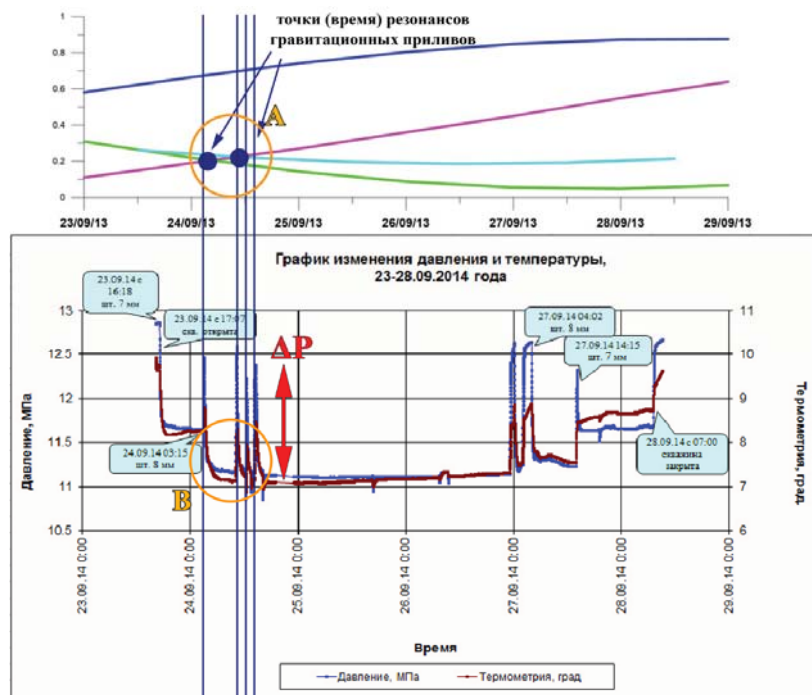
Рис. 15. Колебания давления и температуры в скважине (зона В) под влиянием резонанса приливов (зона А) ( \Delta P \approx 10-15 атм. при P_0 \approx 110 атм. или \Delta P \approx 10-12 % от нормального горного давления)
